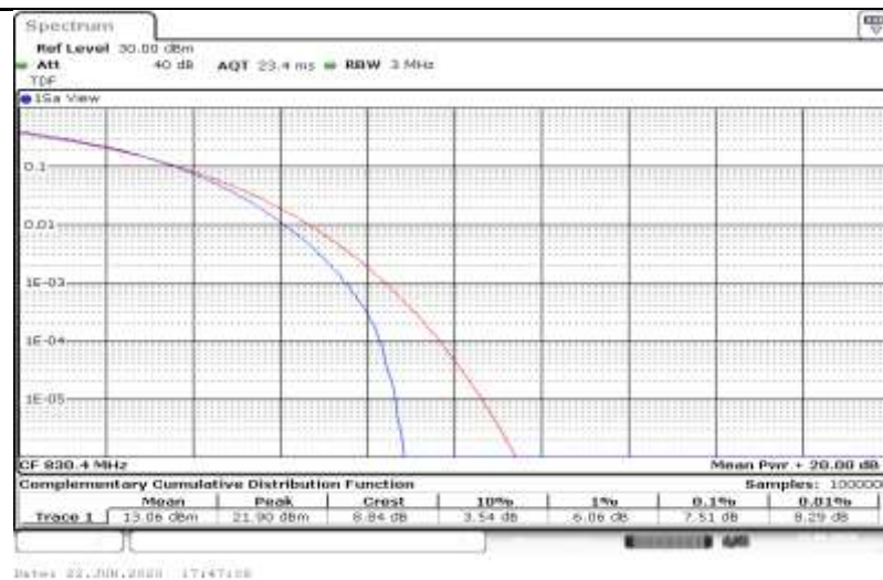
5-5-5MHz-10MHz-QPSK-20478-20550-25RB#0-50RB#0
