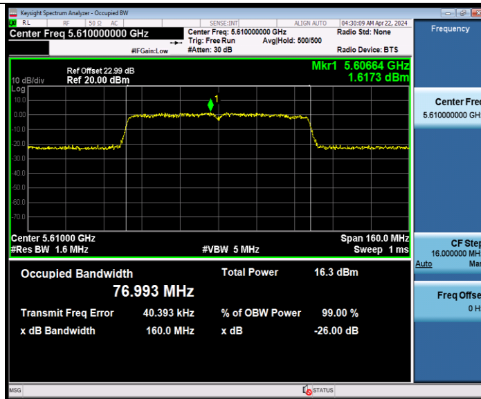
11AC80MIMO_Ant9_5610
