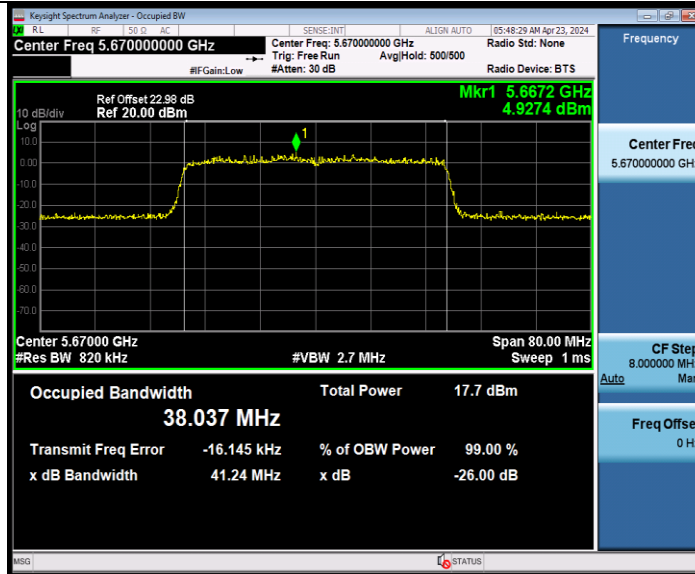
11AX40MIMO_Ant9_5670
