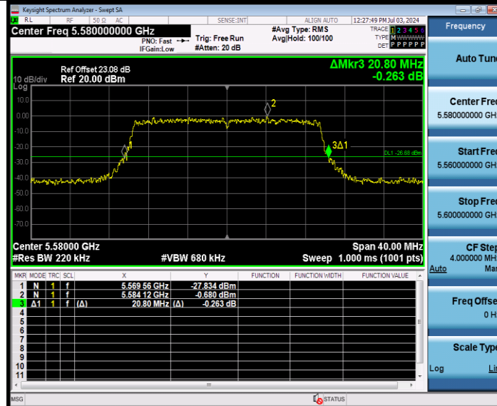
11AX20MIMO_Ant8_5700
