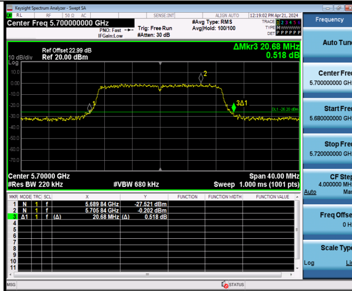
11N20MIMO Ant9 5700
