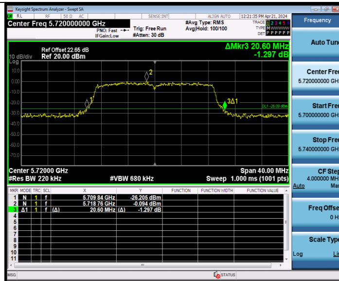
11N20MIMO Ant9 5720
