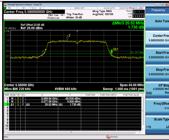
11N20MIMO Ant9 5580
