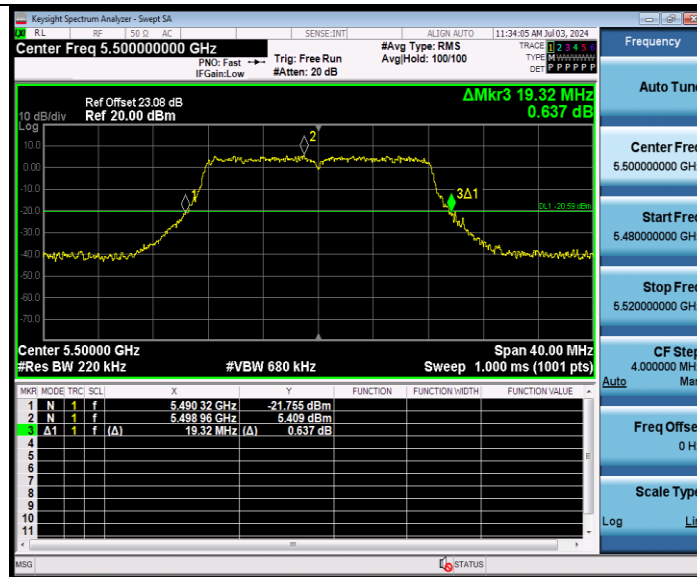
11A-CDD Ant9 5500
