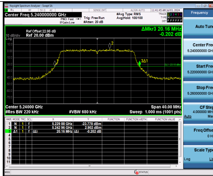
11N20MIMO Ant9 5240
