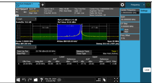
Band48-20MHz-QPSK-55340-1RB#99-PASS
