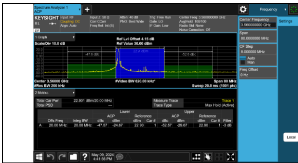
Band48-20MHz-QPSK-55340-1RB#0-PASS
