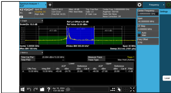
Band48-10MHz-QPSK-56690-1RB#0-PASS
