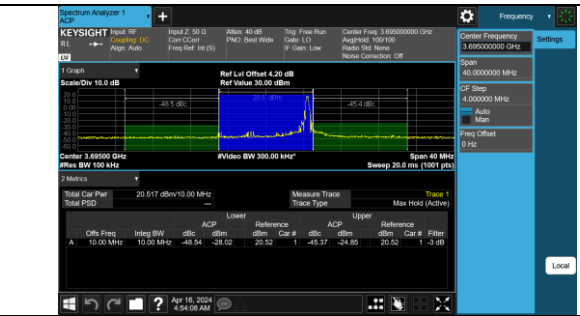
Band48-10MHz-QPSK-56690-1RB#49-PASS
