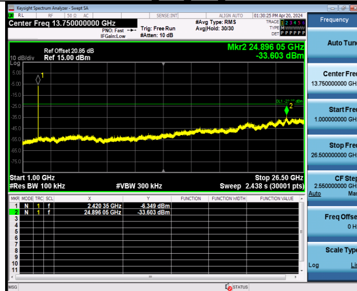
11AX40MIMO_Ant8 2437 0-Reference
