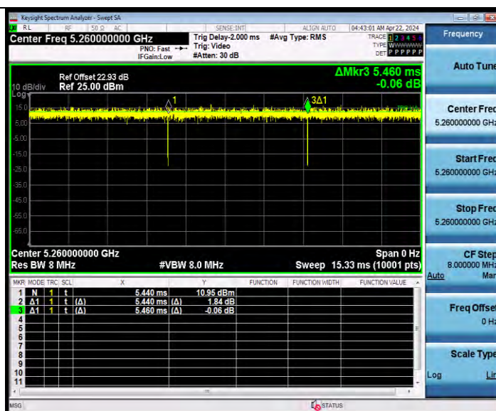
11AX20MIMO_Ant9_5260
