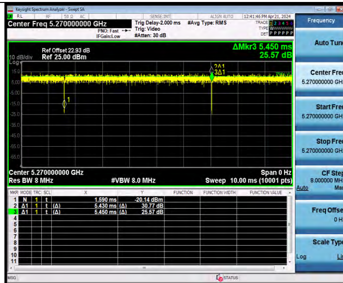
11N40MIMO Ant9 5270
