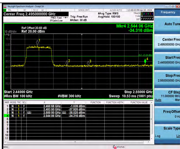
11AX20MIMO_Ant9_High_2462
