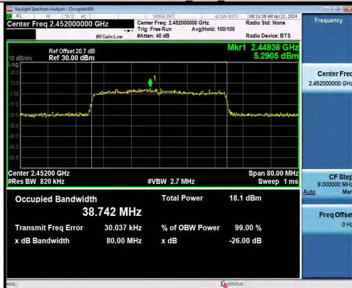
11AX40MIMO_Ant9_2452
