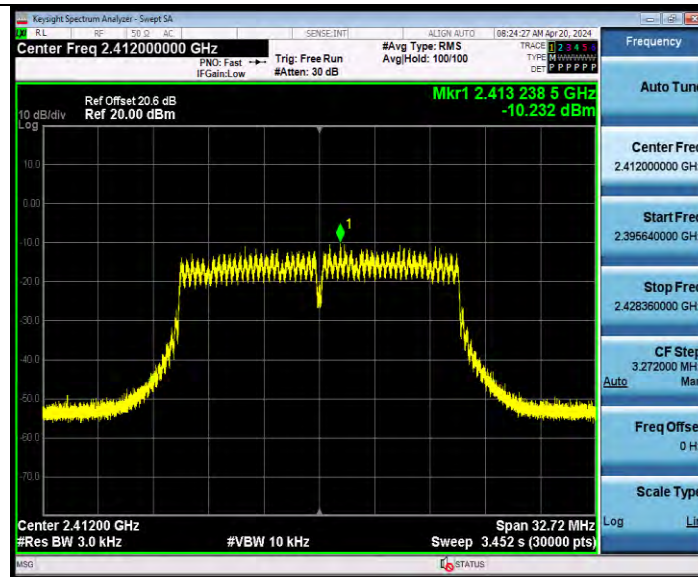
11G-CDD Ant9 2412
