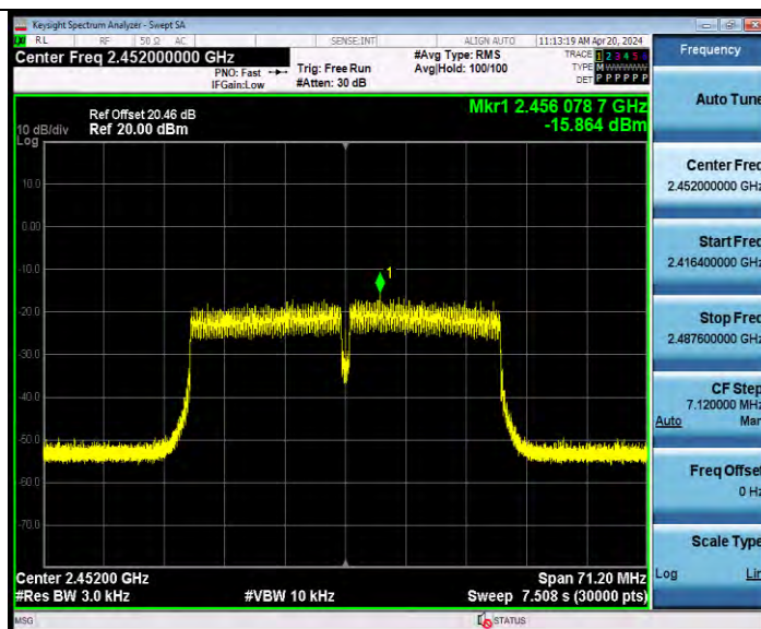
11N40MIMO_Ant9_2452
