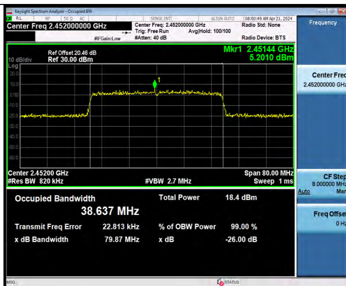
11AX40MIMO_Ant9_2452
