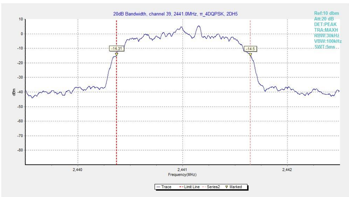
Fig. 82 20dB Bandwidth ( \pi/4 DQPSK, Ch 39)
