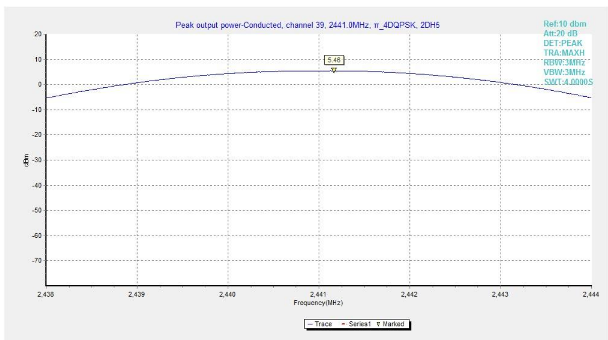
Fig. 5 Peak Output Power ( \pi /4 DQPSK, Ch 39)
