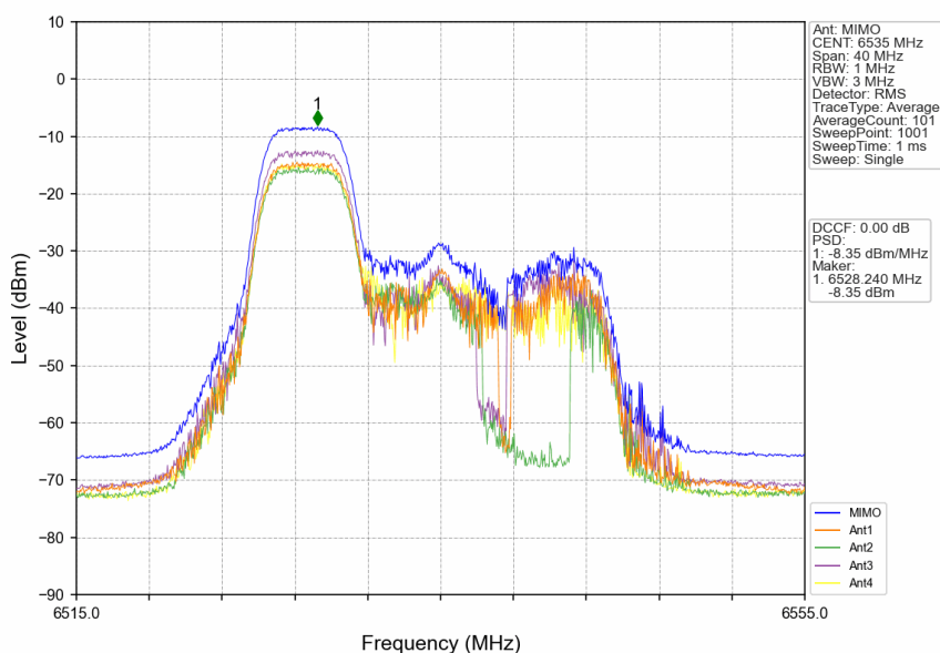
802.11be(EHT20)_LCH_6535MHz_RU52+26_Left_MIMO_NTNV
