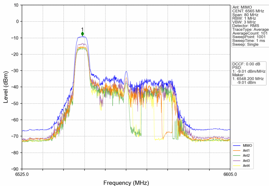
802.11be(EHT40)_LCH_6565MHz_RU52_Left_MIMO_NTNV
