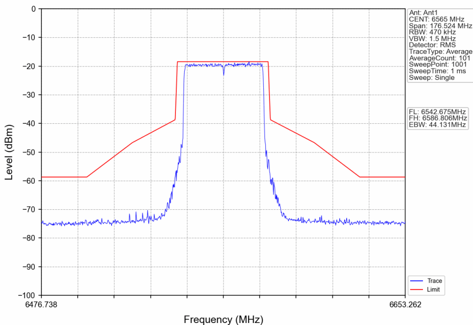
802.11be(EHT40)_LCH_6565MHz_RU484_Left_Ant1_NTNV
