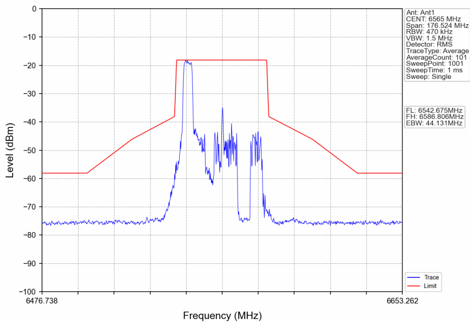
802.11be(EHT40)_LCH_6565MHz_RU52_Left_Ant1_NTNV
