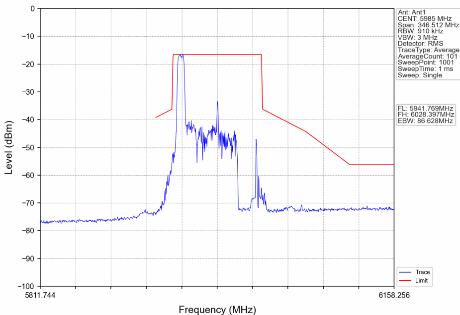
802.11ax(HEW80)_LCH_5985MHz_RU52+26_Left_Ant1_NTNV
