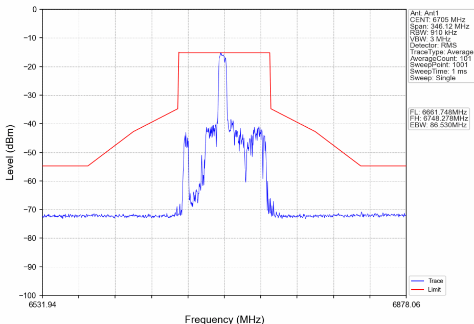
802.11ax(HEW80)_MCH_6705MHz_RU996_Left_Ant1_NTNV
