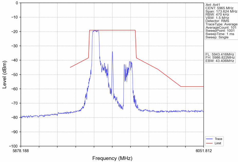
802.11ax(HEW40)_LCH_5965MHz_RU484_Left_Ant1_NTNV
