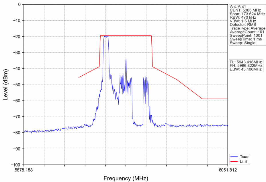
802.11ax(HEW40)_LCH_5965MHz_RU52_Left_Ant1_NTNV
