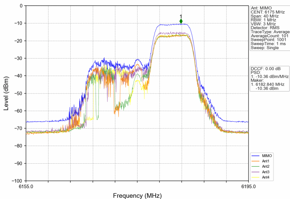
802.11be(EHT20)_MCH_6175MHz_RU242_Left_MIMO_NTNV
