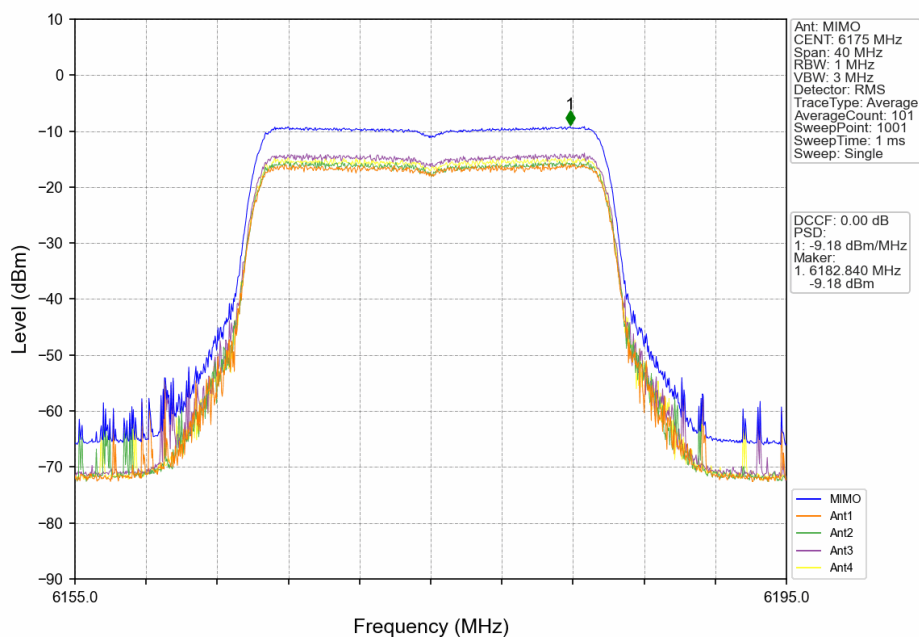
802.11be(EHT20)_MCH_6175MHz_RU242_Left_MIMO_NTNV
