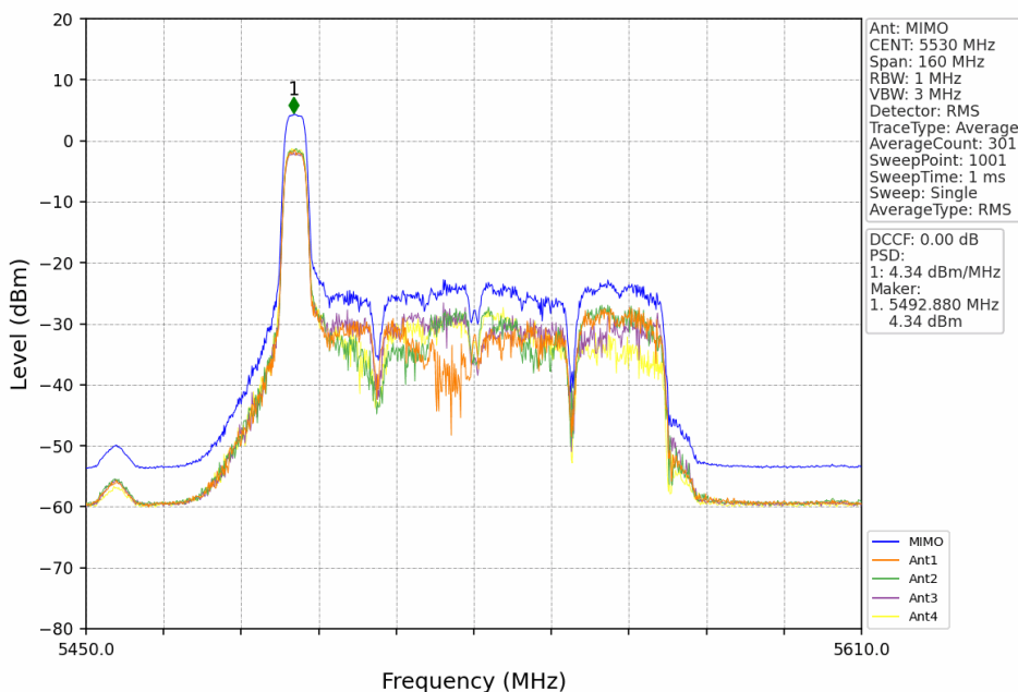
802.11be(EHT80)_LCH_5530MHz_RU52_Left_MIMO_NTNV
