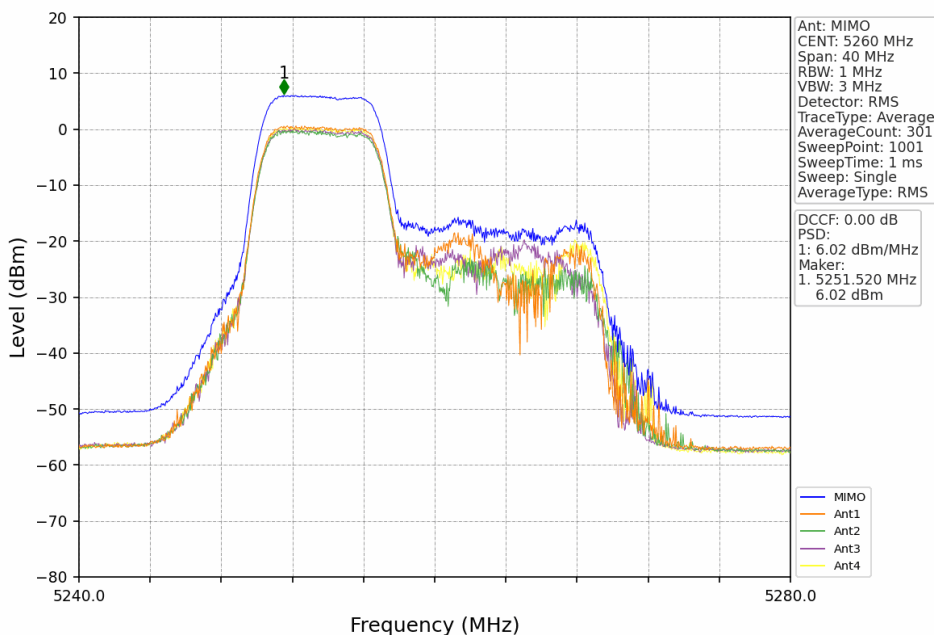
802.11be(EHT20)_LCH_5260MHz_RU52_Left_MIMO_NTNV
