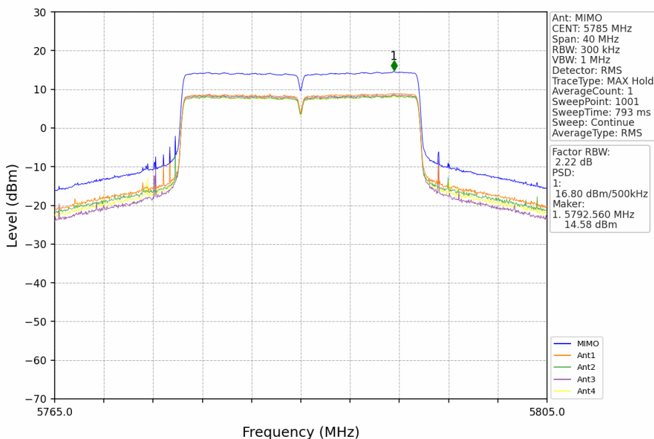
802.11be(EHT20)_MCH_5785MHz_RU242_Left_MIMO_NTNV
