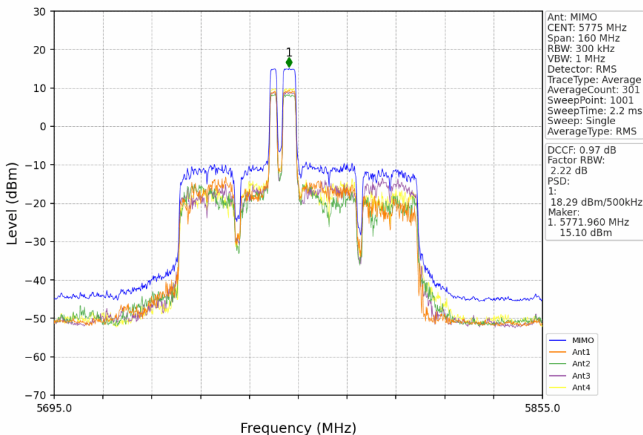
802.11be(EHT80)_MCH_5775MHz_RU996_Left_MIMO_NTNV
