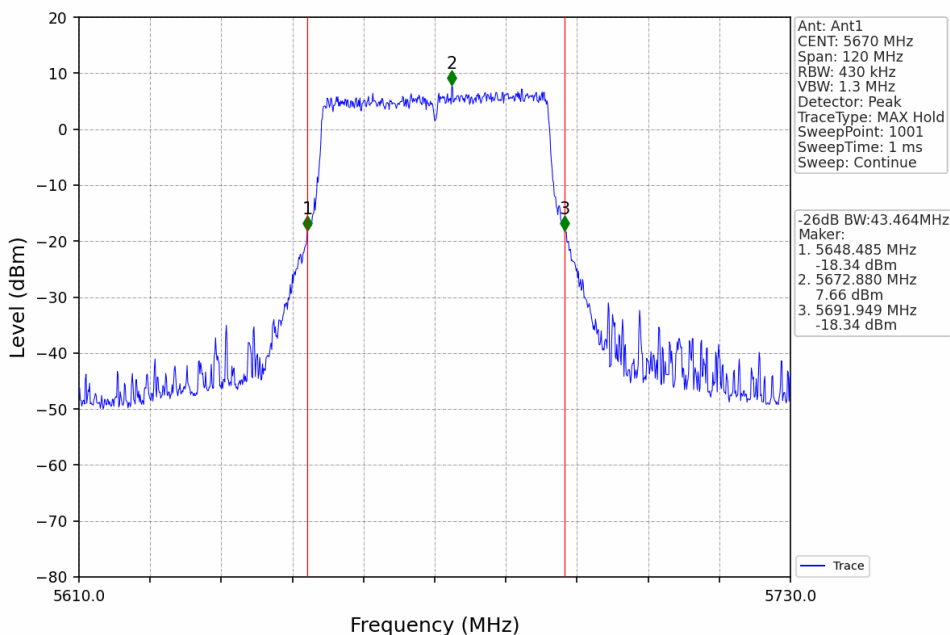
802.11ax(HEW40)_HCH_5670MHz_RU484_Left_Ant1_NTNV
