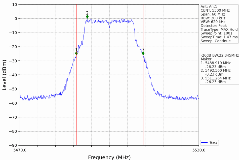
802.11a_LCH_5500MHz_Ant1_NTNV
