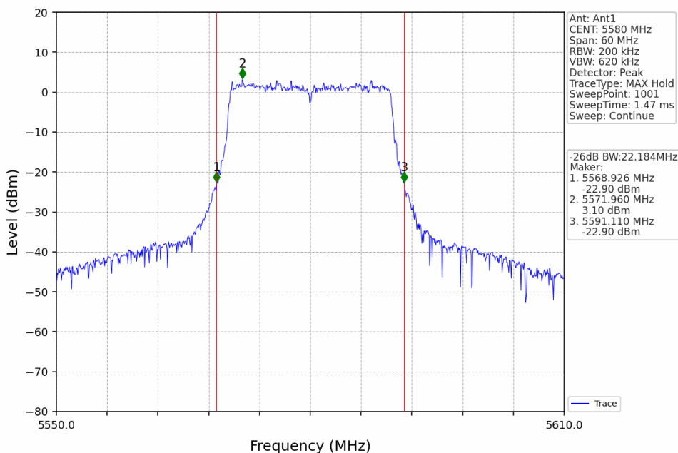
802.11be(EHT20)_MCH_5580MHz_RU242_Left_Ant1_NTNV
