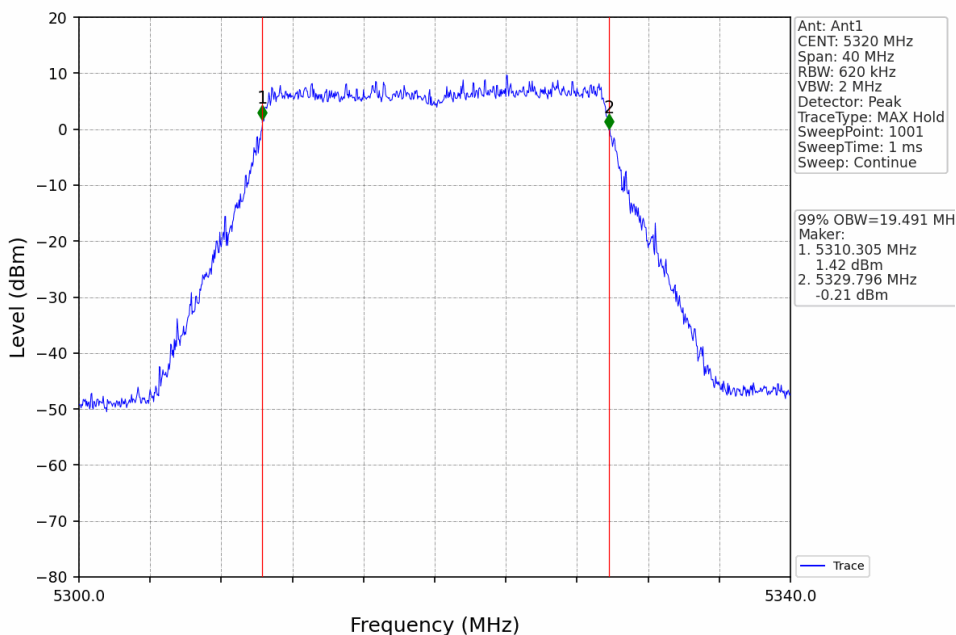
802.11ax(HEW20)_HCH_5320MHz_RU242_Left_Ant1_NTNV
