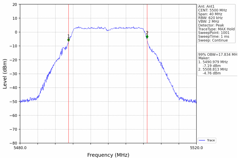
802.11a_LCH_5500MHz_Ant1_NTNV
