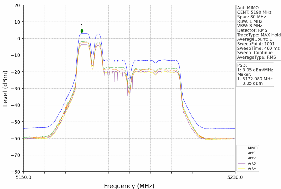
802.11be(EHT40)_LCH_5190MHz_RU52+26_Left_MIMO_NTNV
