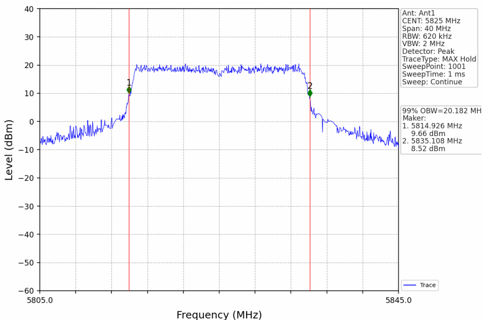
802.11be(EHT20)_HCH_5825MHz_RU242_Left_Ant1_NTNV
