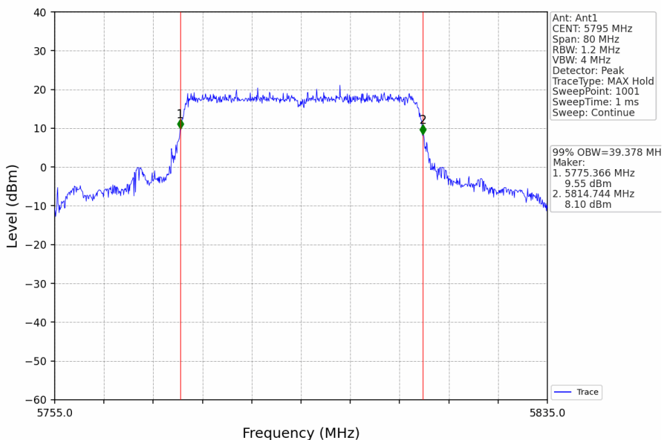
802.11be(EHT40)_HCH_5795MHz_RU484_Left_Ant1_NTNV
