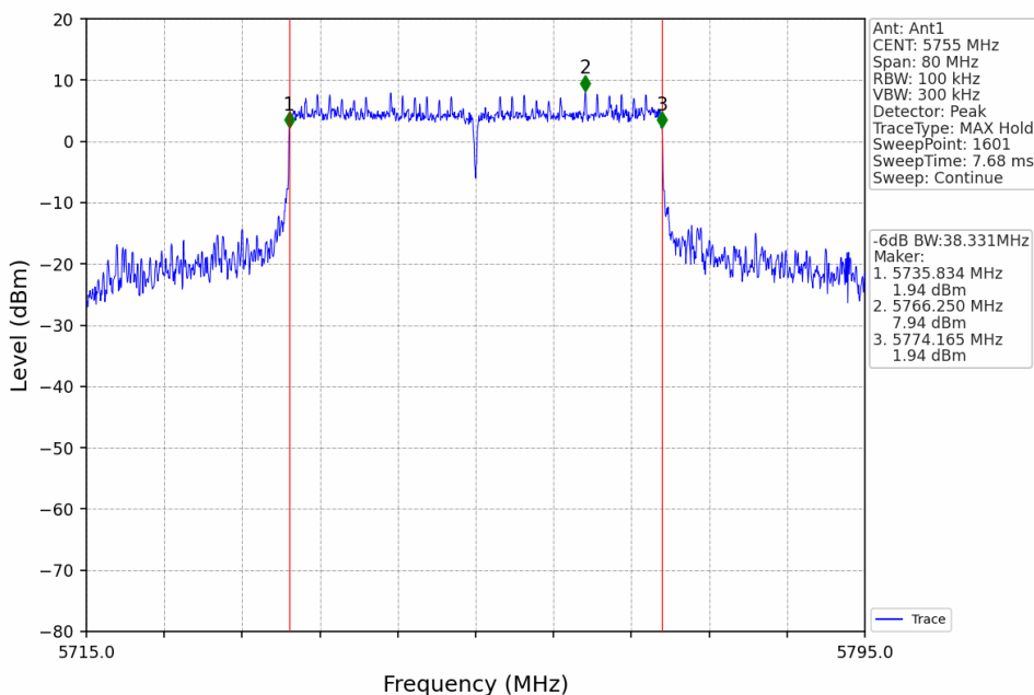
802.11be(EHT40)_LCH_5755MHz_RU484_Left_Ant1_NTNV
