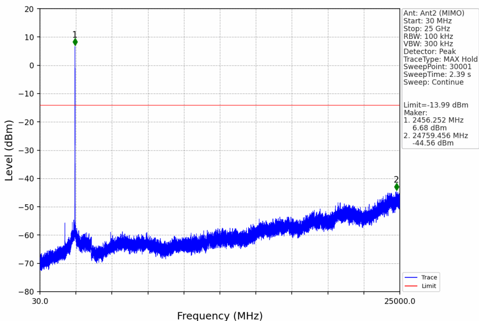
802.11ax(HEW20)_HCH_2462MHz_RU52_Left_Ant2 (MIMO)_NTNV
