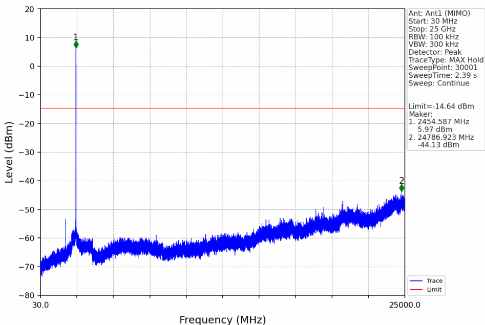
802.11ax(HEW20)_HCH_2462MHz_RU52_Left_Ant1 (MIMO)_NTNV
