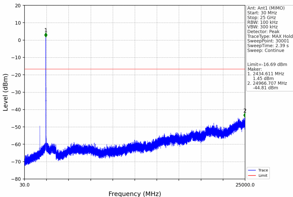
802.11ax(HEW40)_HCH_2452MHz_RU52_Left_Ant1 (MIMO)_NTNV
