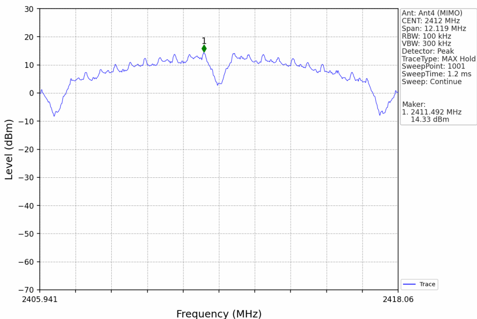
802.11b_LCH_2412MHz_Ant4 (MIMO)_NTNV
