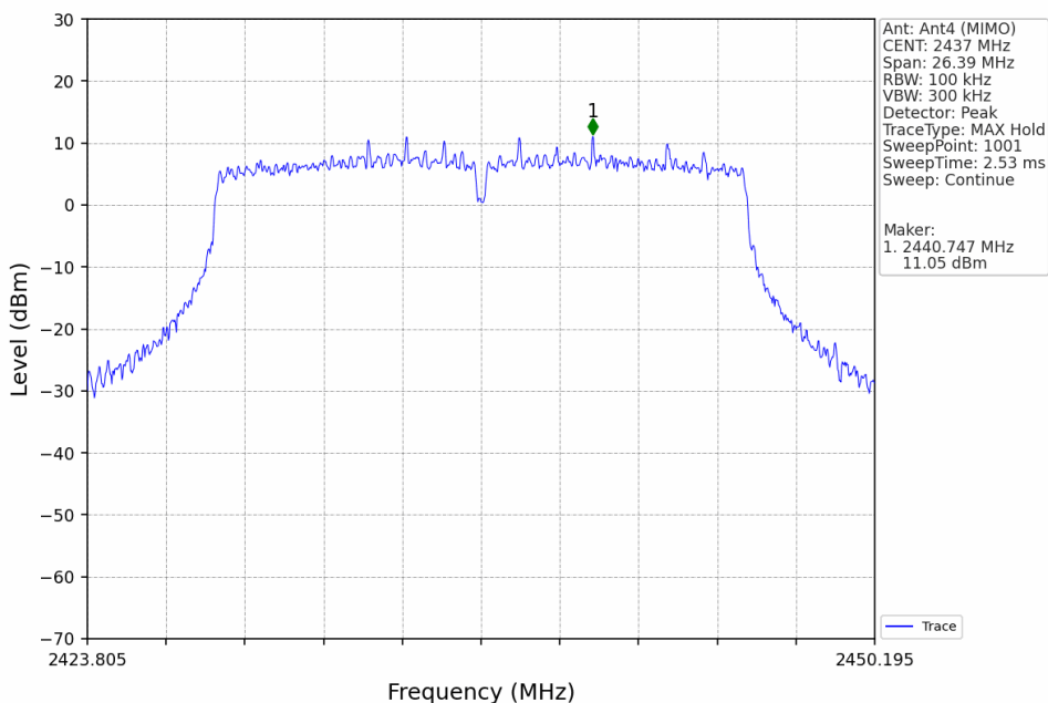
802.11n(HT20)_MCH_2437MHz_Ant4 (MIMO)_NTNV
