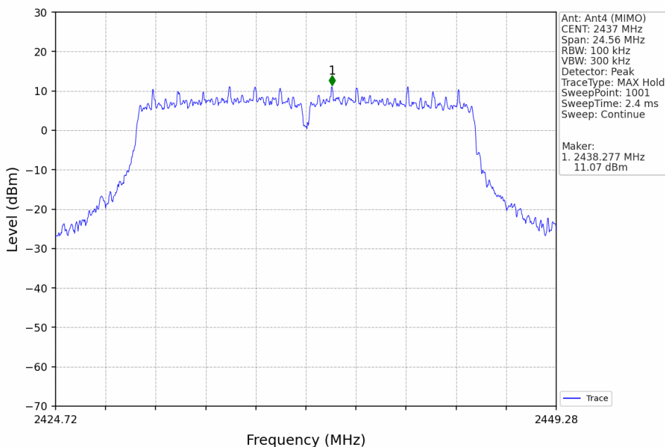
802.11g_MCH_2437MHz_Ant4 (MIMO)_NTNV
