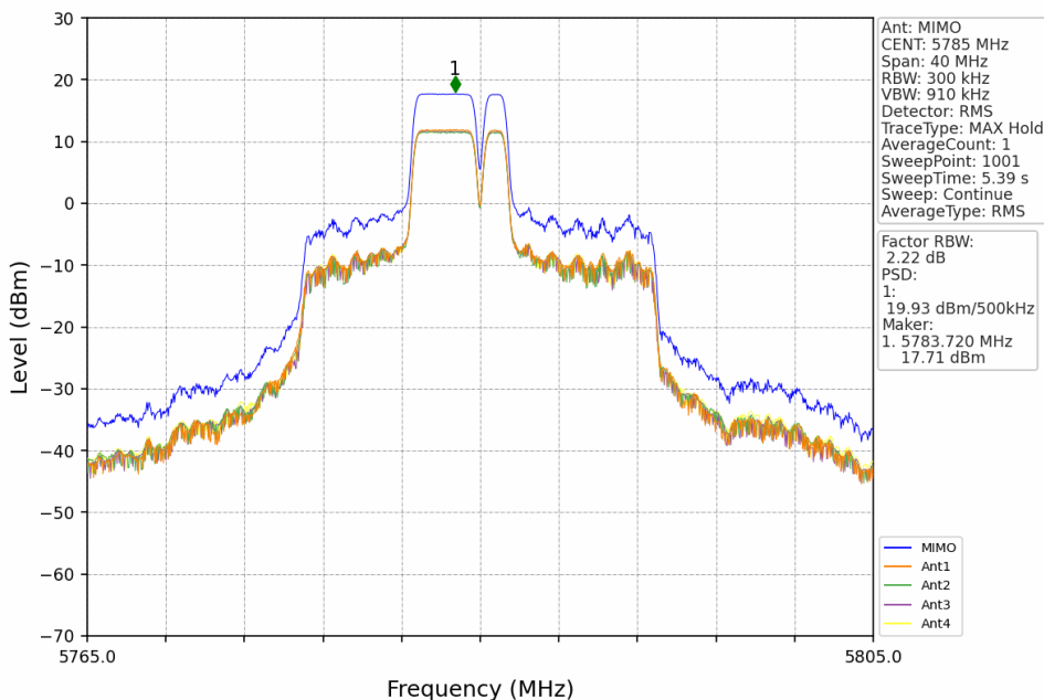
802.11ax(HEW20) MCH 5785MHz RU52 Mid MIMO NTN
