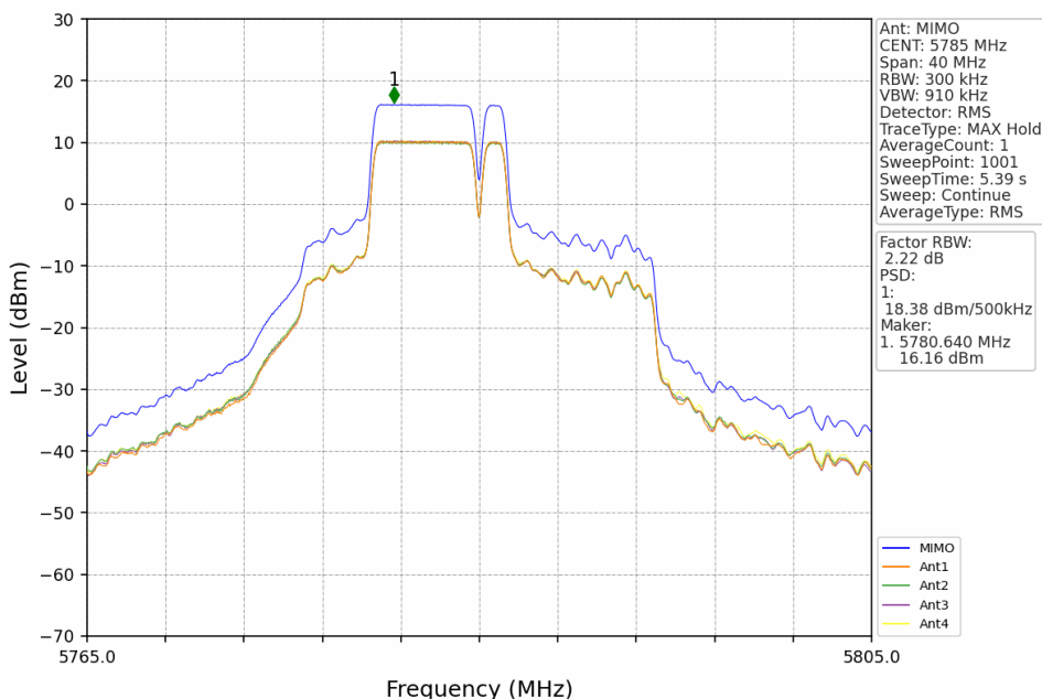
802.11be(EHT20) MCH 5785MHz RU242 Left MIMO NTN
