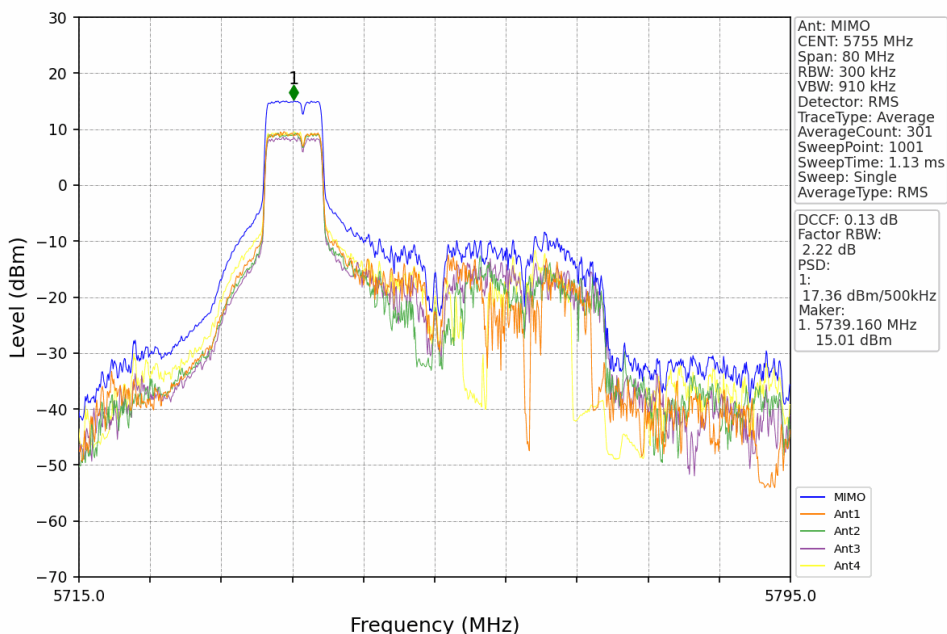
802.11ax(HEW40) LCH 5755MHz RU484 Left MIMO NTN
