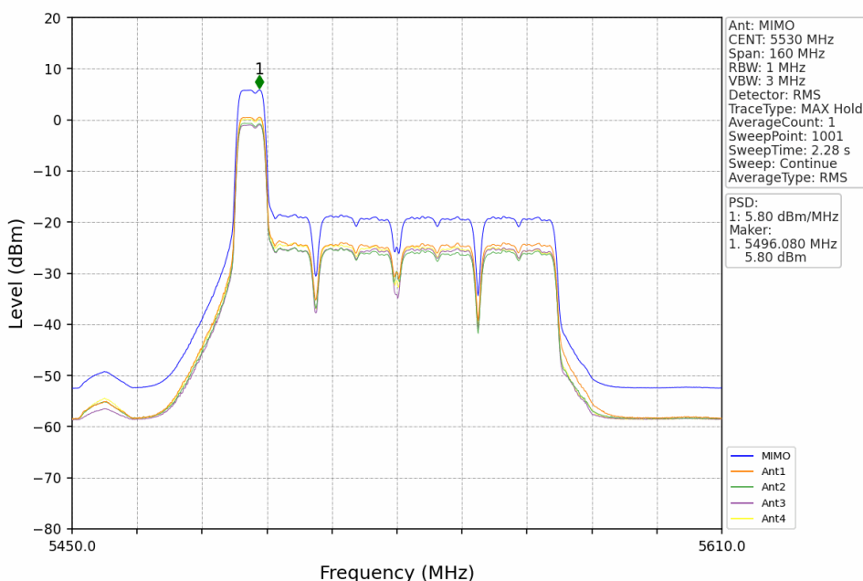
802.11be(EHT80) LCH 5530MHz RU996 Left MIMO NTN
