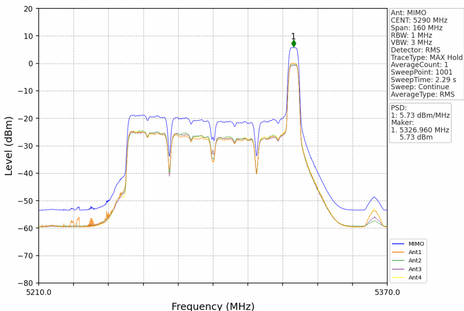
802.11be(EHT80)_MCH_5290MHz_RU52+26_Right_MIMO_NTNV
