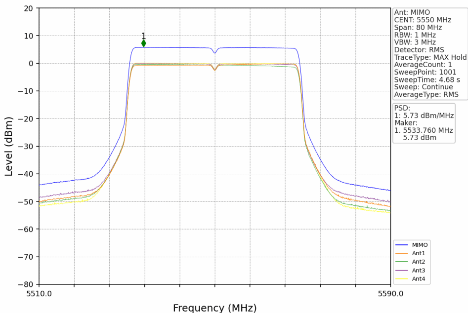
802.11be(EHT40) MCH 5550MHz RU484 Left MIMO NTN
