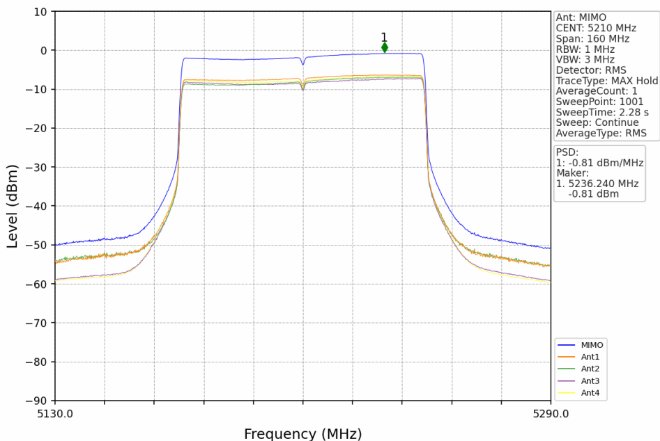
802.11be(EHT80) MCH 5210MHz RU996 Left MIMO NTN
