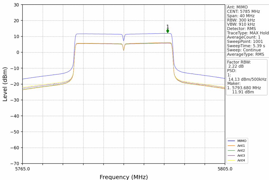
802.11ax(HEW20) MCH 5785MHz RU242 Left MIMO NTN
