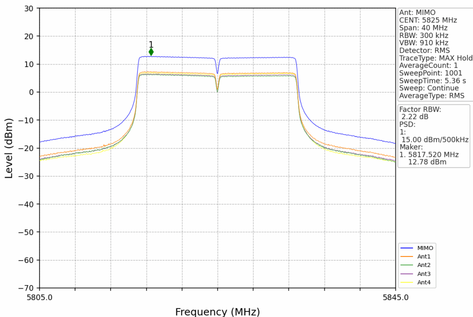
802.11n(HT20) HCH 5825MHz MIMO NTN
