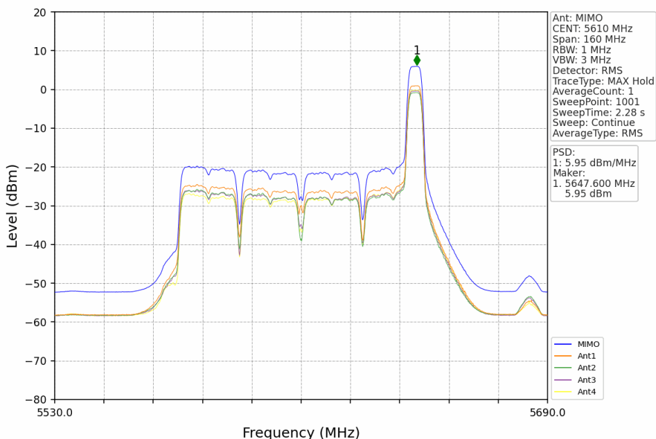
802.11be(EHT80)_HCH_5610MHz_RU52+26_Right_MIMO_NTNV
