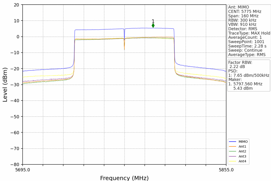
802.11ax(HEW80) MCH 5775MHz RU996 Left MIMO NTN
