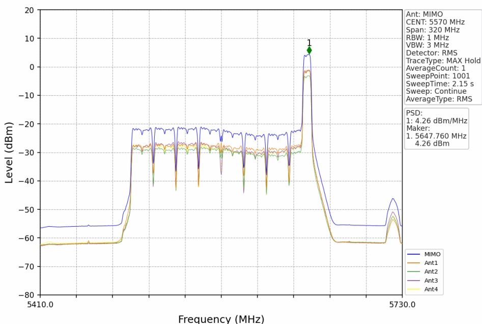
802.11be(EHT160) MCH 5570MHz 2xRU996 Left MIMO NTN
