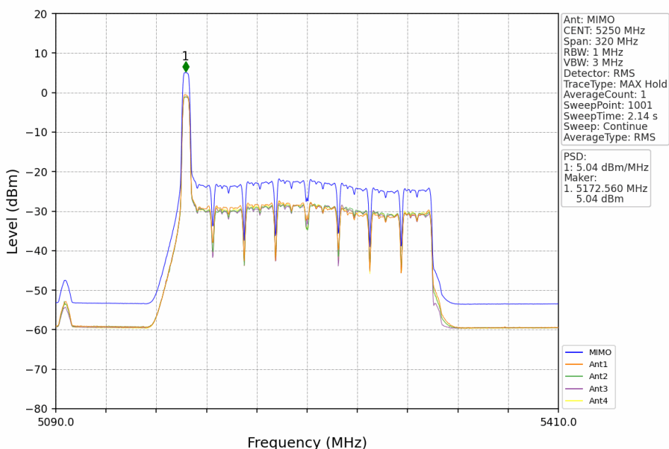
802.11be(EHT160) MCH 5250MHz RU52+26 Left MIMO_NTNV
