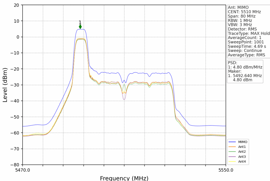
802.11be(EHT40) LCH 5510MHz RU52+26 Left MIMO NTN
