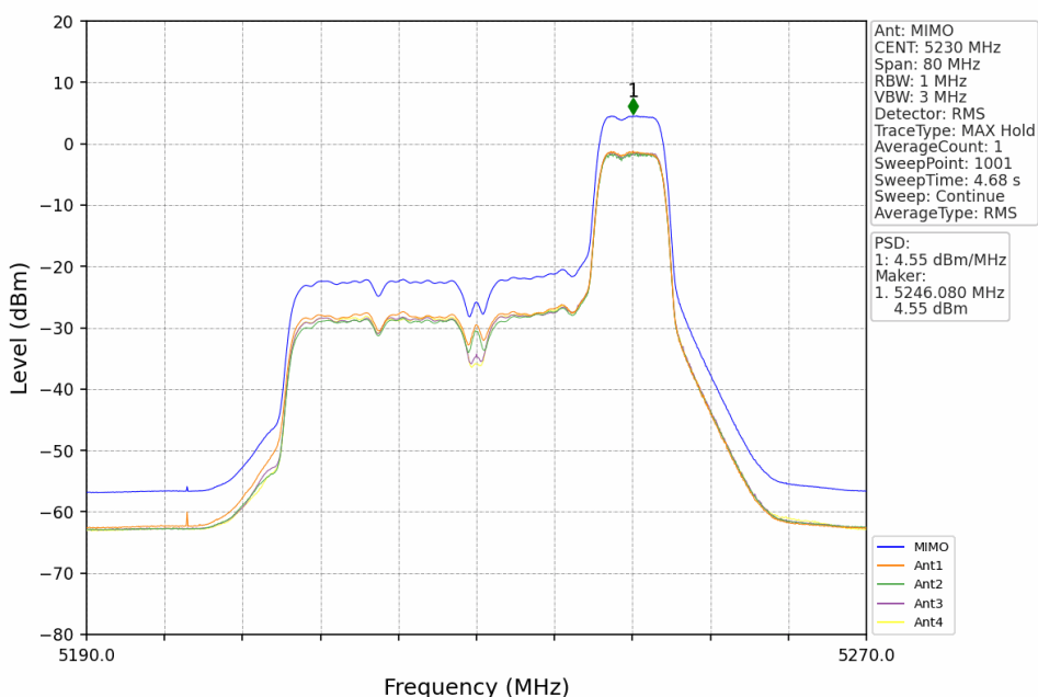
802.11be(EHT40)_HCH_5230MHz_RU484_Left_MIMO_NTNV
