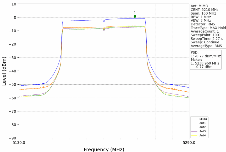
802.11ax(HEW80) MCH 5210MHz RU996 Left MIMO NTN
