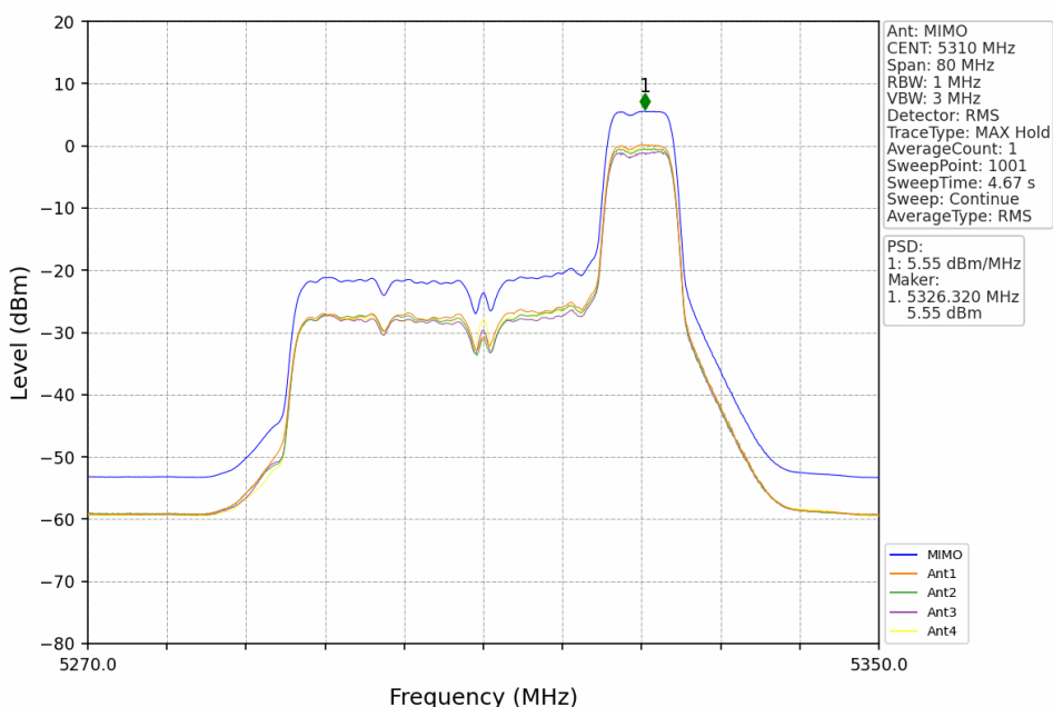
802.11ax(HEW40) HCH 5310MHz RU484 Left MIMO NTN
