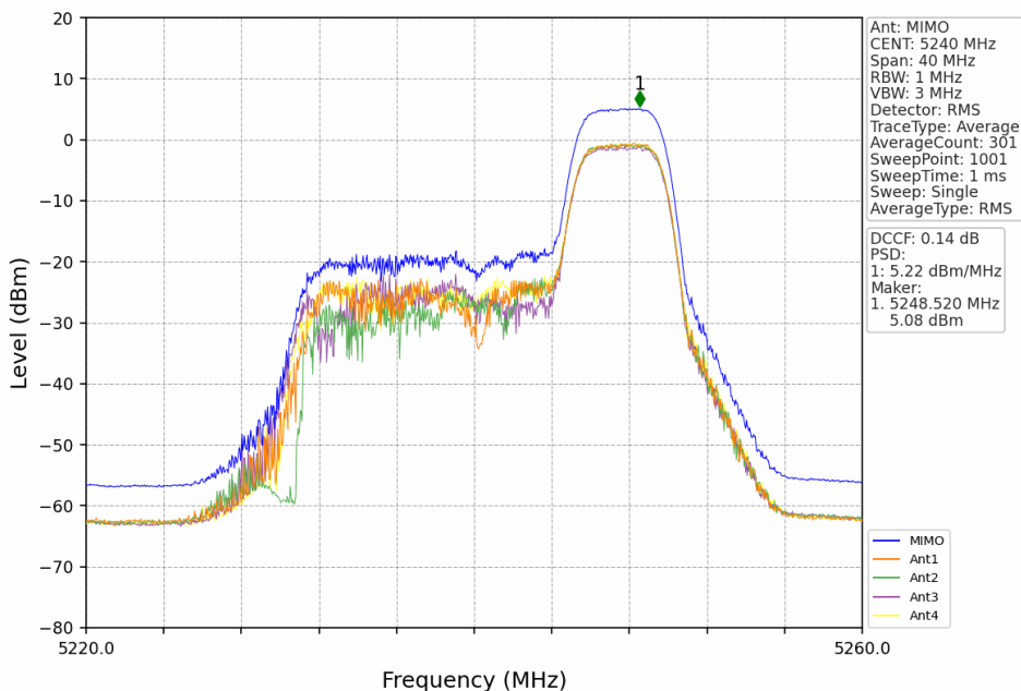
802.11be(EHT20) HCH 5240MHz RU52 Right MIMO NTN
