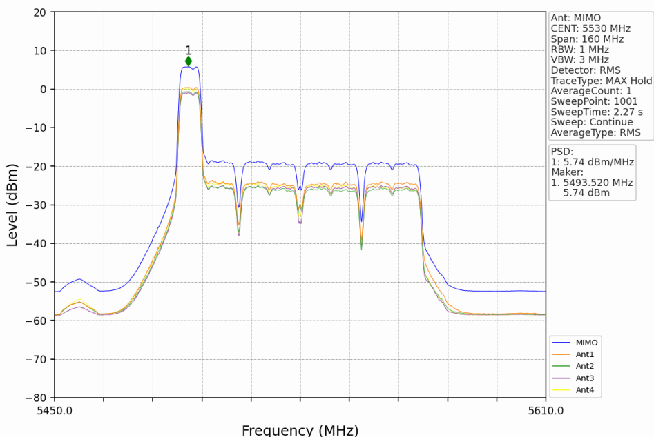
802.11ax(HEW80) LCH 5530MHz RU996 Left MIMO NTNv
