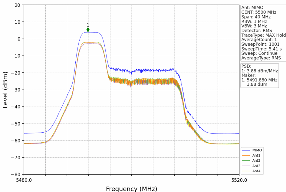
802.11be(EHT20)_LCH_5500MHz_RU52_Left_MIMO_NTNV
