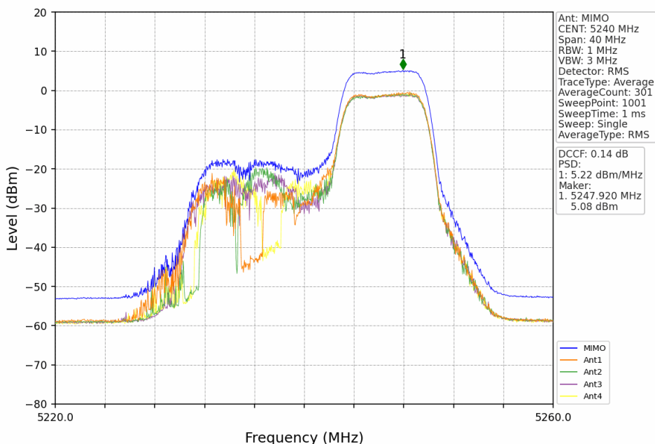
802.11be(EHT20)_HCH_5240MHz_RU242_Left_MIMO_NTNV
