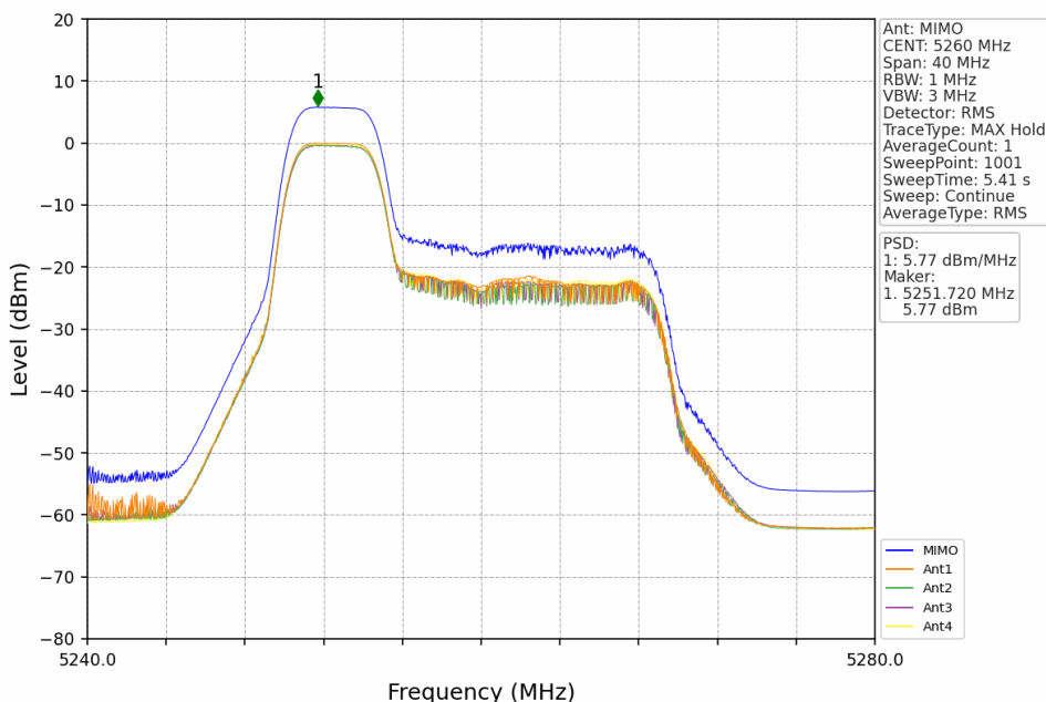
802.11be(EHT20) LCH 5260MHz RU52+26 Left MIMO NTN
