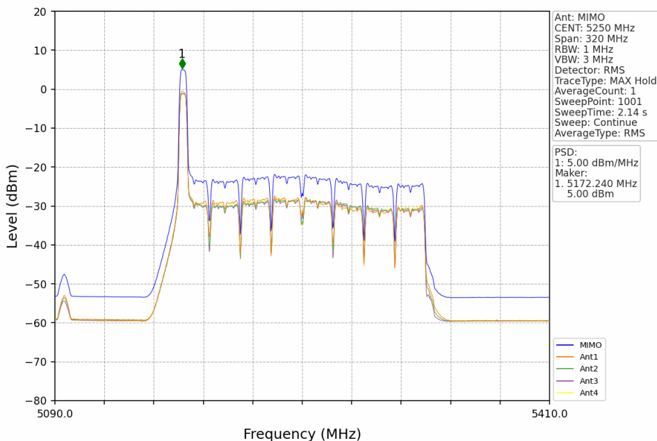
802.11ax(HEW160) MCH 5250MHz RU52+26 Left MIMO NTNV
