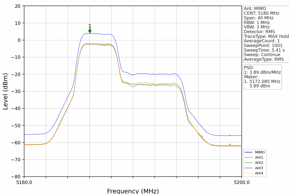
802.11be(EHT20) LCH 5180MHz RU242 Left MIMO NTN
