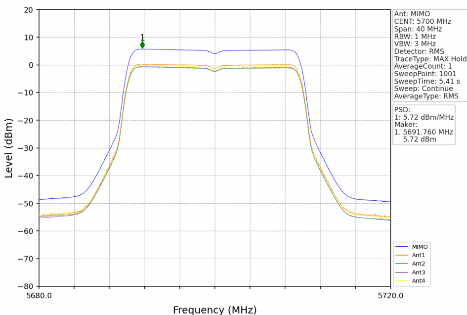
802.11be(EHT20) HCH 5700MHz RU242 Left MIMO NTNV
