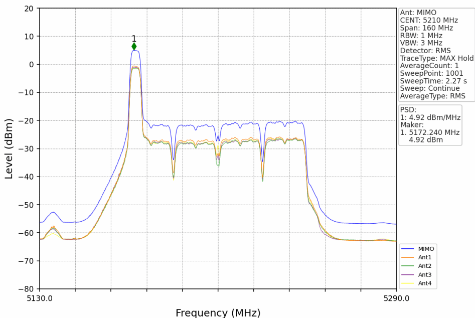
802.11ax(HEW80) MCH 5210MHz RU52 Left MIMO NTN
