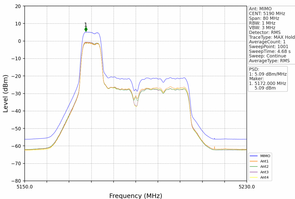
802.11be(EHT40) LCH 5190MHz RU52+26 Left MIMO NTN
