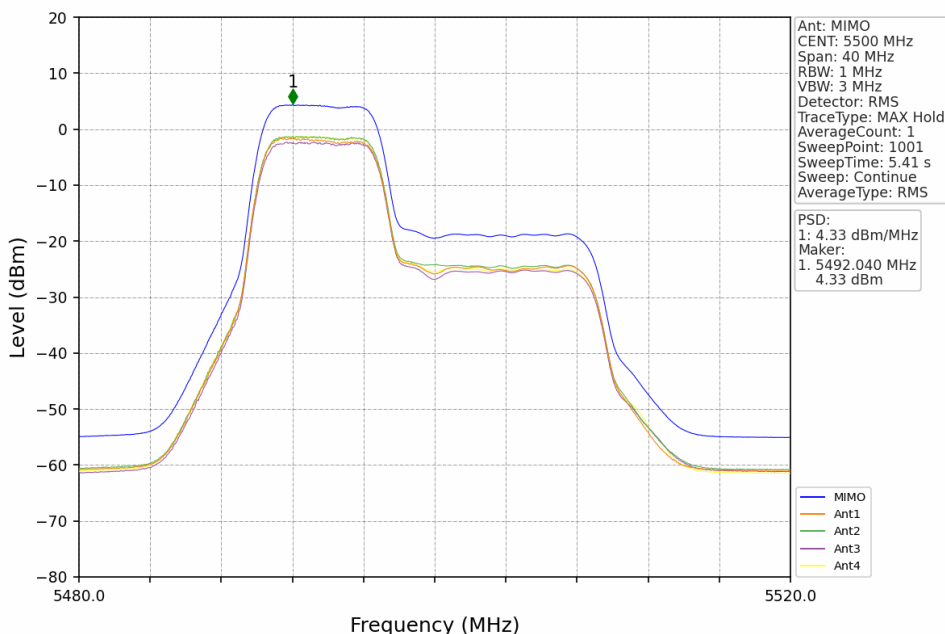
802.11be(EHT20) LCH 5500MHz RU242 Left MIMO NTN
