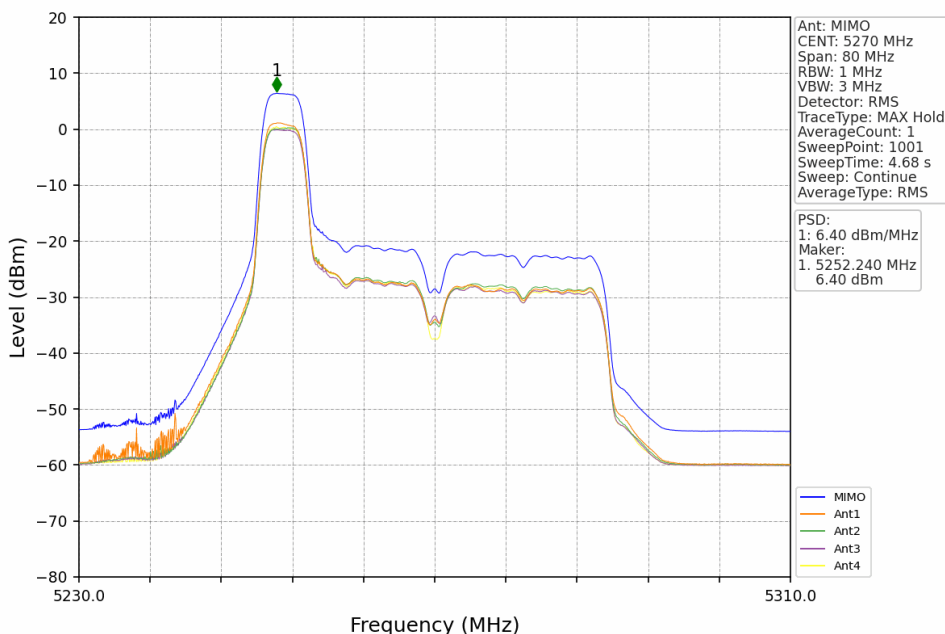
802.11be(EHT40) LCH 5270MHz RU52+26 Left MIMO NTN
