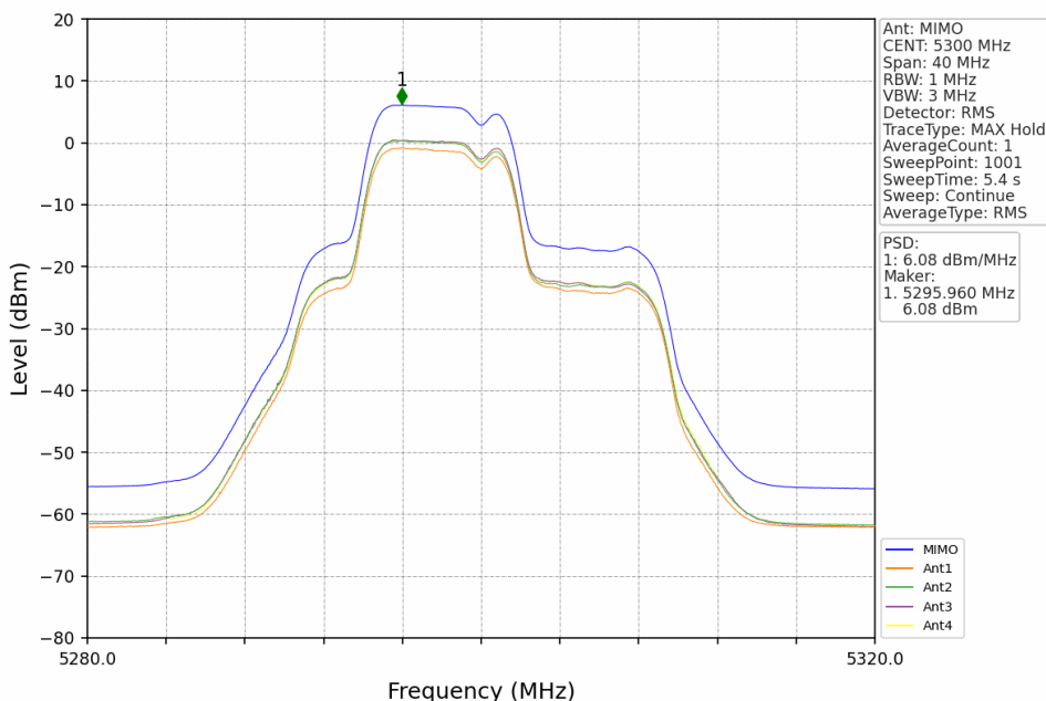
802.11ax(HEW20) MCH 5300MHz RU242 Left MIMO NTN
