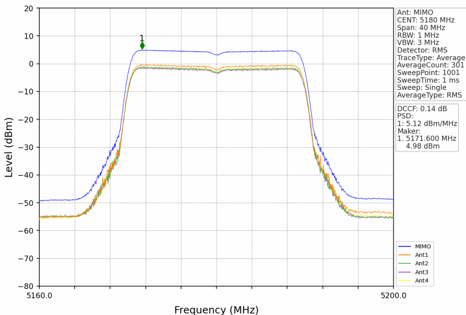
802.11ax(HEW20) LCH 5180MHz RU242 Left MIMO NTN
