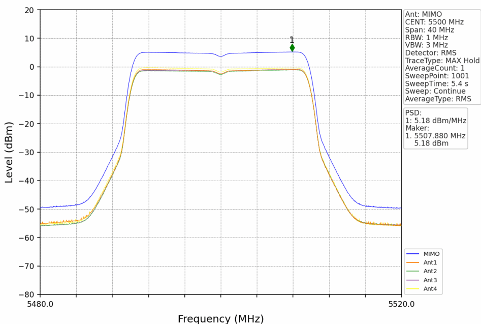
802.11ax(HEW20) LCH 5500MHz RU242 Left MIMO NTNv
