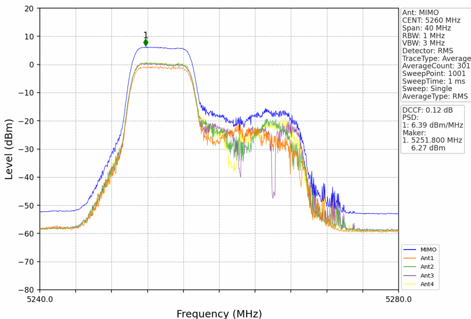
802.11ax(HEW20) LCH 5260MHz RU52+26 Left MIMO NTN
