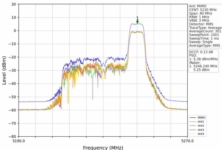
802.11ax(HEW40) HCH 5230MHz RU484 Left MIMO NTN
