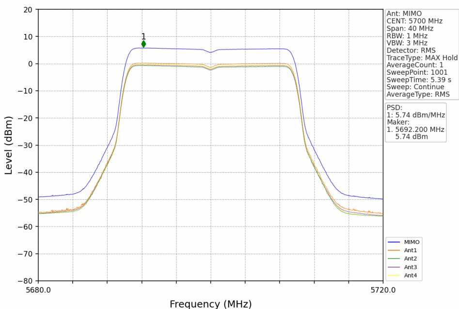
802.11ax(HEW20) HCH 5700MHz RU242 Left MIMO NTN
