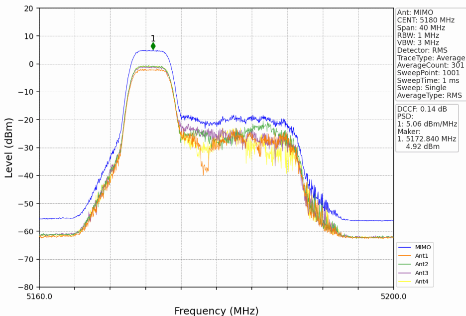
802.11ax(HEW20) LCH 5180MHz RU52 Left MIMO NTN
