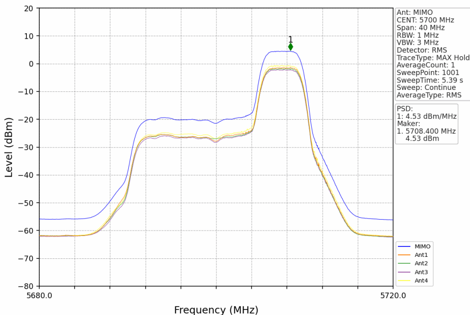
802.11ax(HEW20) HCH 5700MHz RU52 Right MIMO NTN
