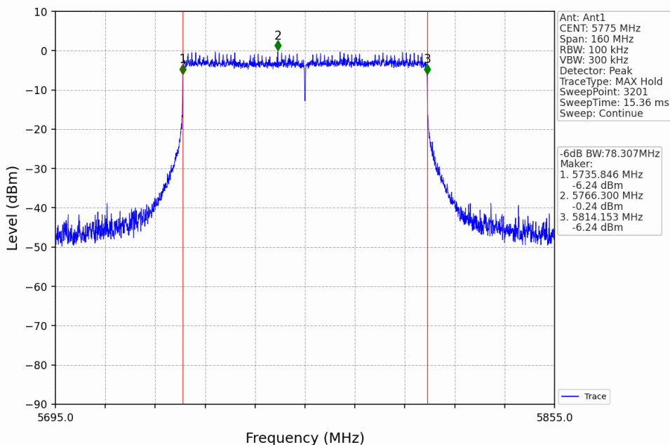
802.11be(EHT80)_MCH_5775MHz_RU996_Left_Ant1_NTNV
