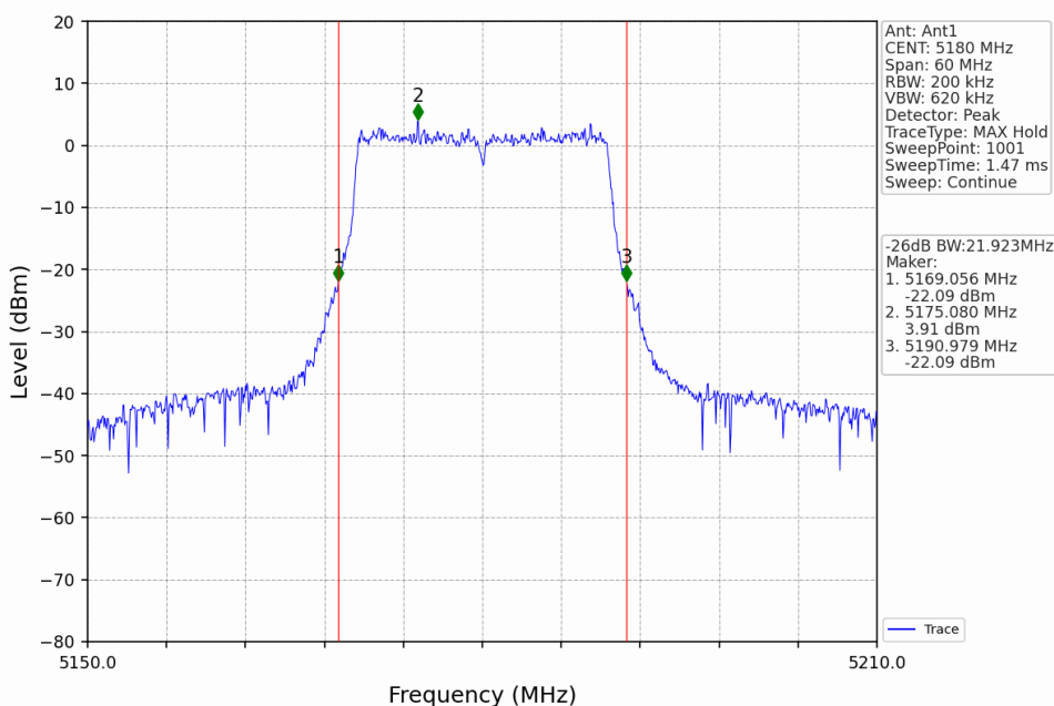
802.11be(EHT20) LCH_5180MHz_RU242_Left_Ant1_NTNV
