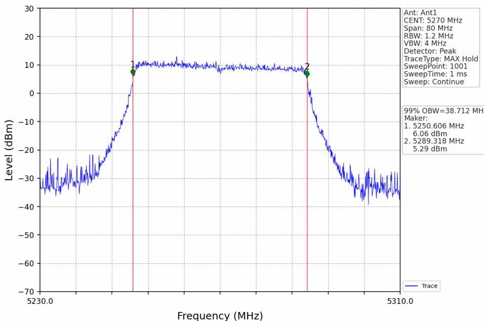
802.11ax(HEW40) LCH 5270MHz RU484 Left Ant1 NTN
