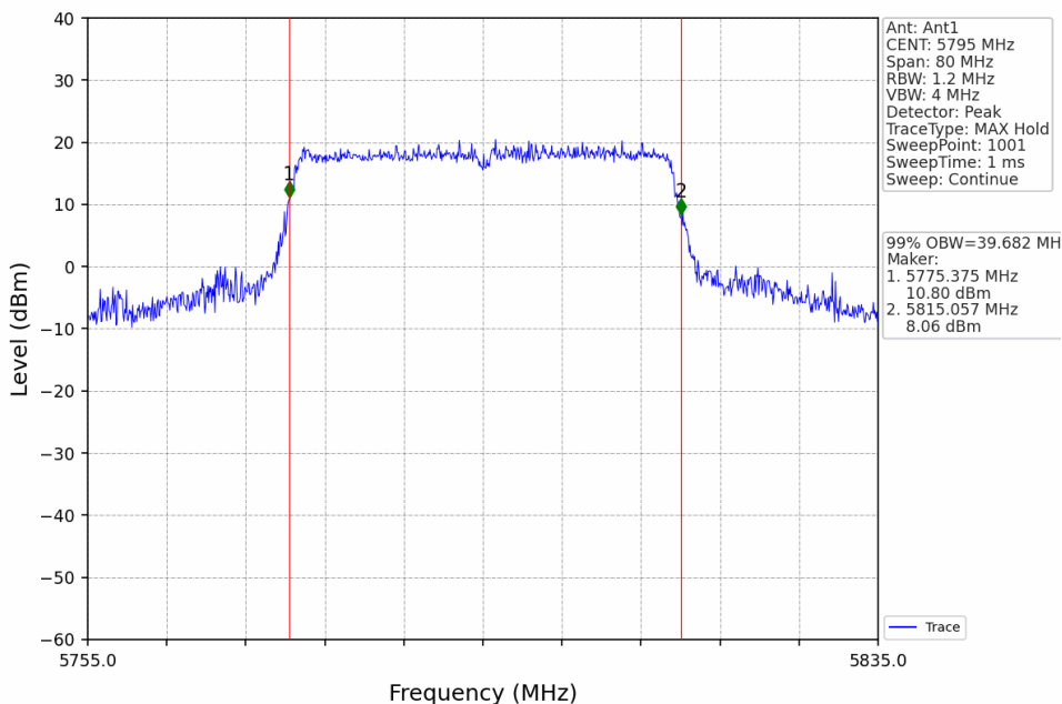
802.11be(EHT40) HCH_5795MHz RU484 Left Ant1 NTVN
