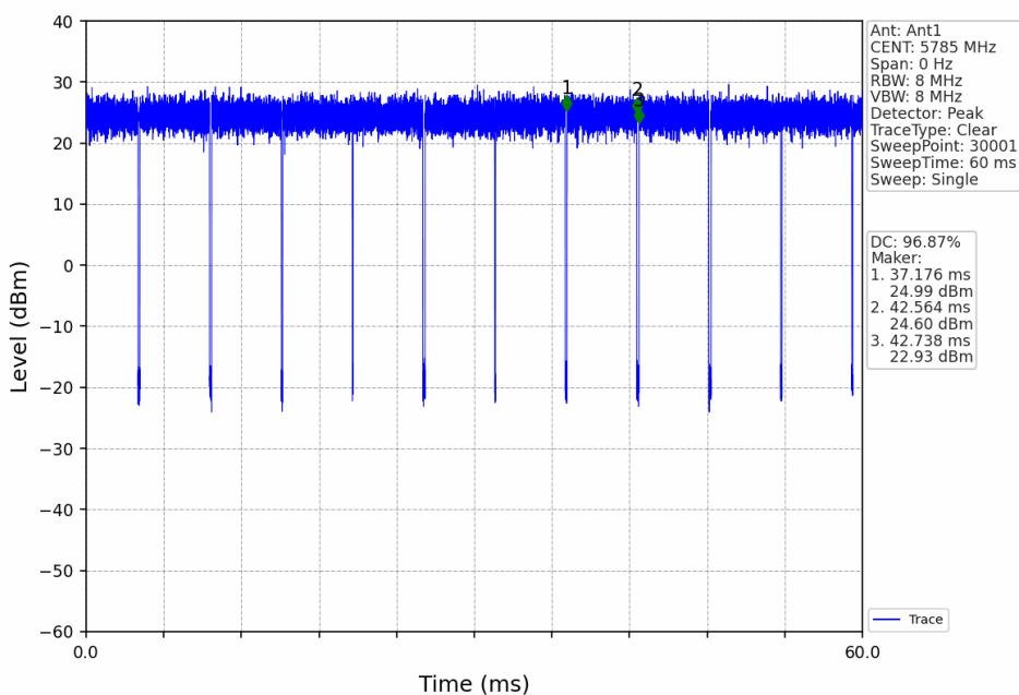
802.11be(EHT20)_MCH_5785MHz_RU242_Left_Ant1_NTNV
