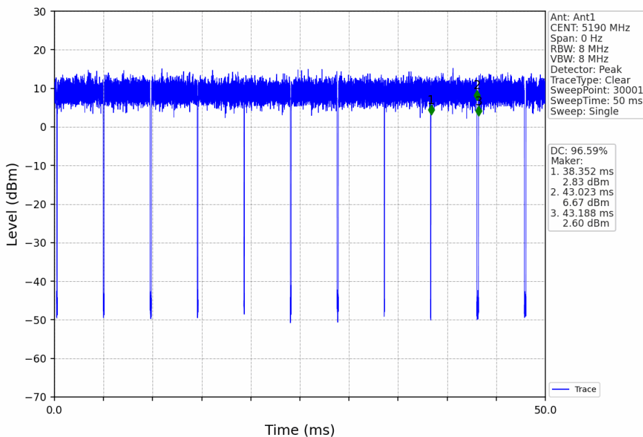
802.11be(EHT40)_LCH_5190MHz_RU484_Left_Ant1_NTNV
