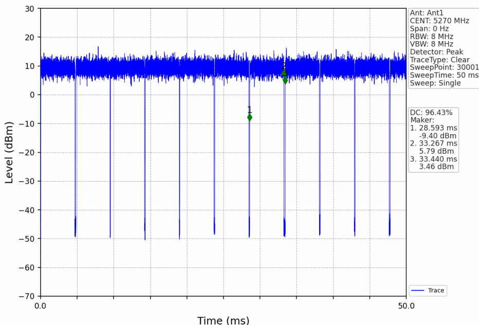
802.11be(EHT40)_LCH_5270MHz_RU484_Left_Ant1_NTNV
