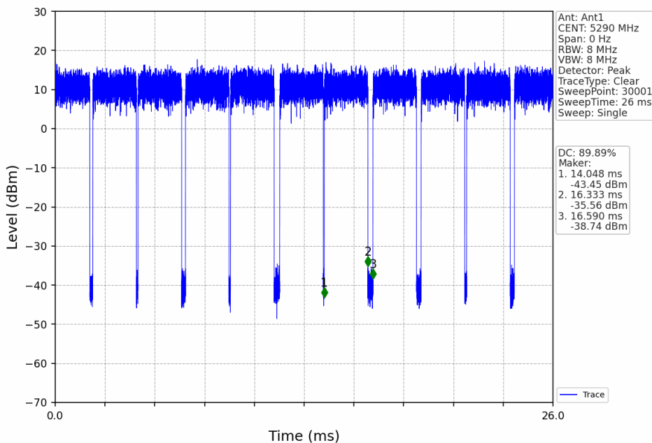
802.11be(EHT80)_MCH_5290MHz_RU996_Left_Ant1_NTNV
