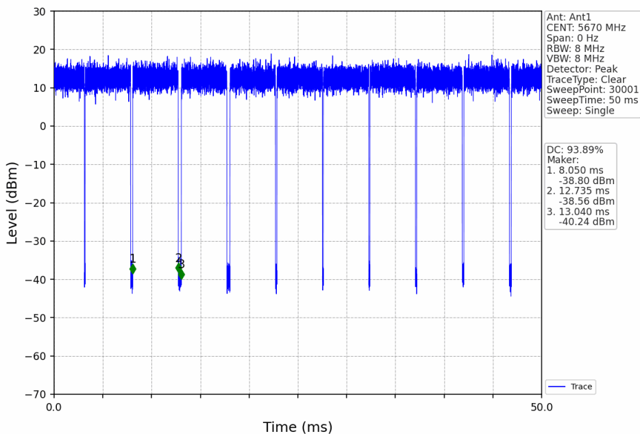
802.11be(EHT40)_HCH_5670MHz_RU484_Left_Ant1_NTNV
