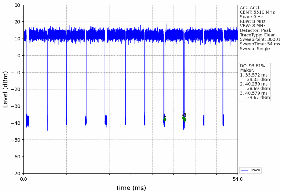
802.11be(EHT40)_LCH_5510MHz_RU484_Left_Ant1_NTNV
