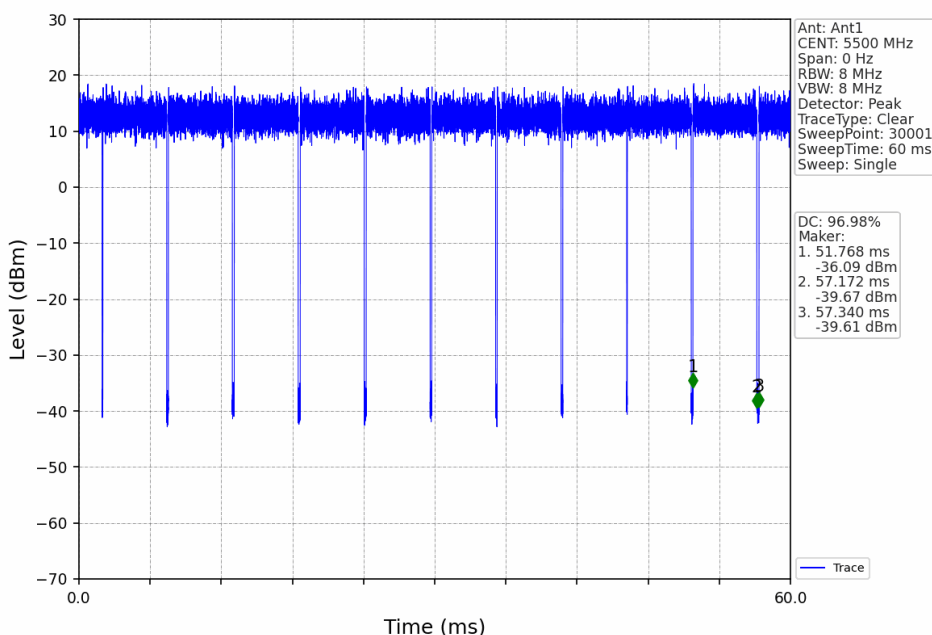
802.11be(EHT20)_LCH_5500MHz_RU242_Left_Ant1_NTNV
