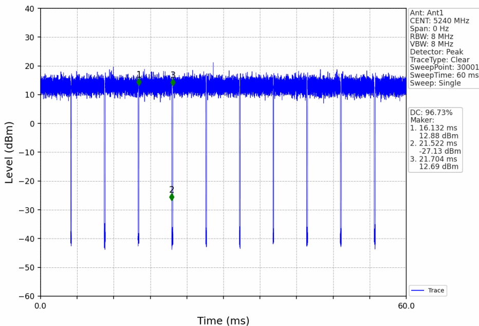
802.11be(EHT20)_HCH_5240MHz_RU242_Left_Ant1_NTNV
