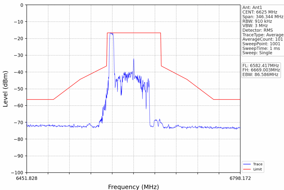
802.11ax(HEW80) LCH 6625MHz RU52+26 Left Ant1 NTNV
