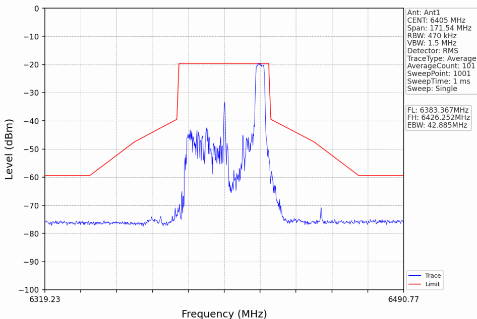
802.11ax(HEW40) HCH 6405MHz RU52 Right Ant1 NTN
