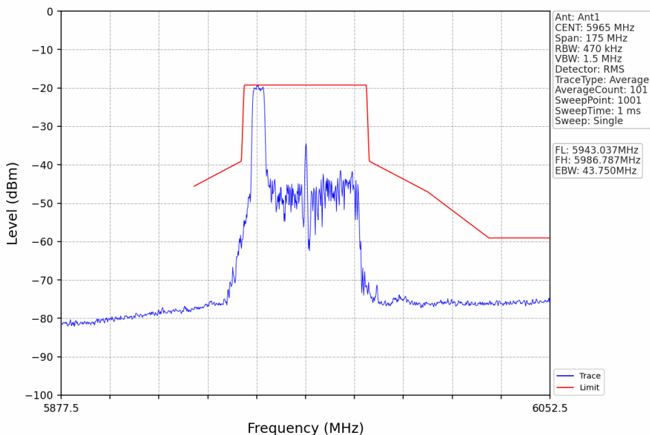
802.11ax(HEW40) LCH 5965MHz RU52 Left Ant1 NTN
