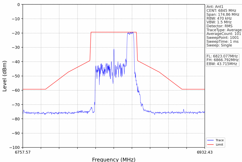
802.11ax(HEW40) HCH 6845MHz RU484 Left Ant1 NTVN
