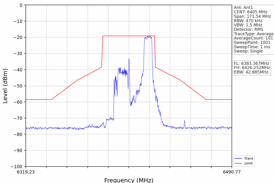
802.11ax(HEW40) HCH 6405MHz RU484 Left Ant1 NTVN
