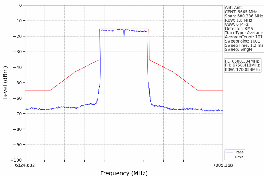
802.11ax(HEW160) MCH 6665MHz 2xRU996 Left Ant1 NTVN
