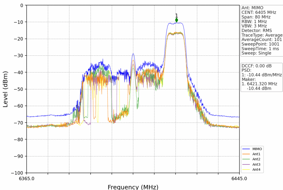
802.11ax(HEW40) HCH 6405MHz RU484 Left MIMO NTN
