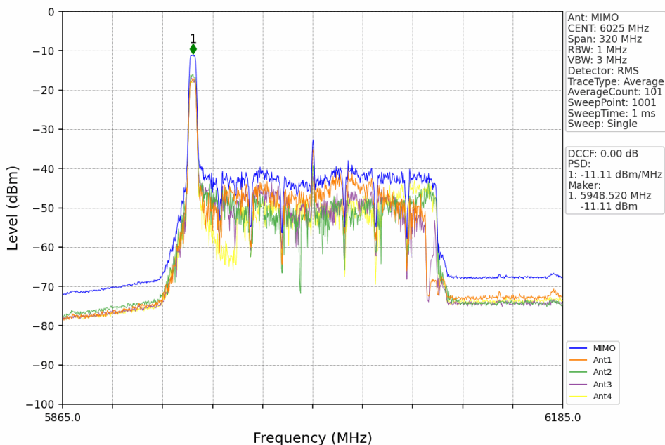
802.11ax(HEW160) LCH 6025MHz RU52 Left MIMO NTN
