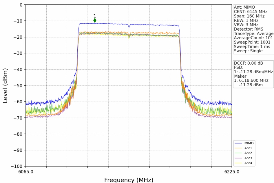
802.11ax(HEW80) MCH 6145MHz RU996 Left MIMO NTN
