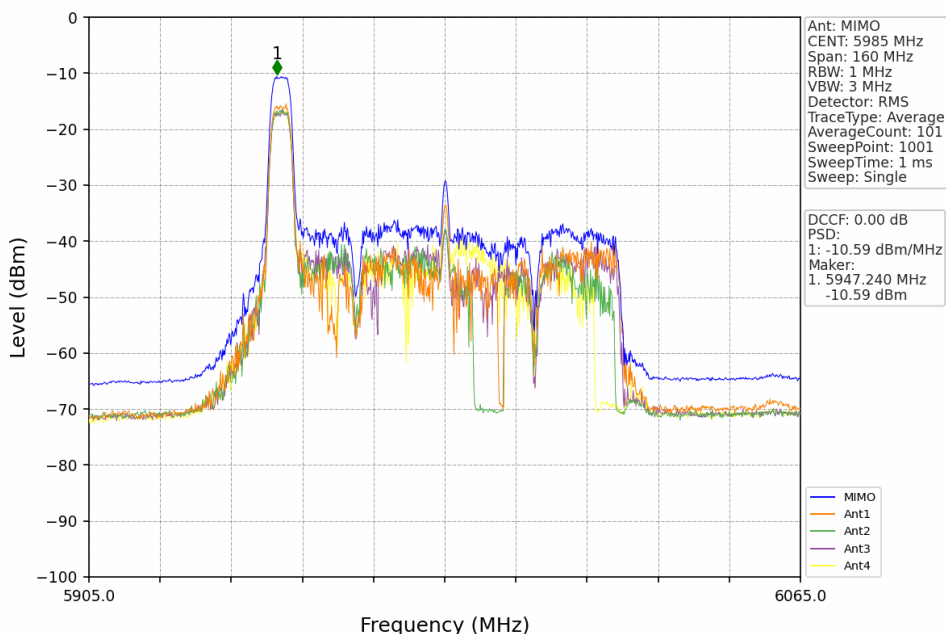
802.11ax(HEW80) LCH 5985MHz RU52+26 Left MIMO NTN
