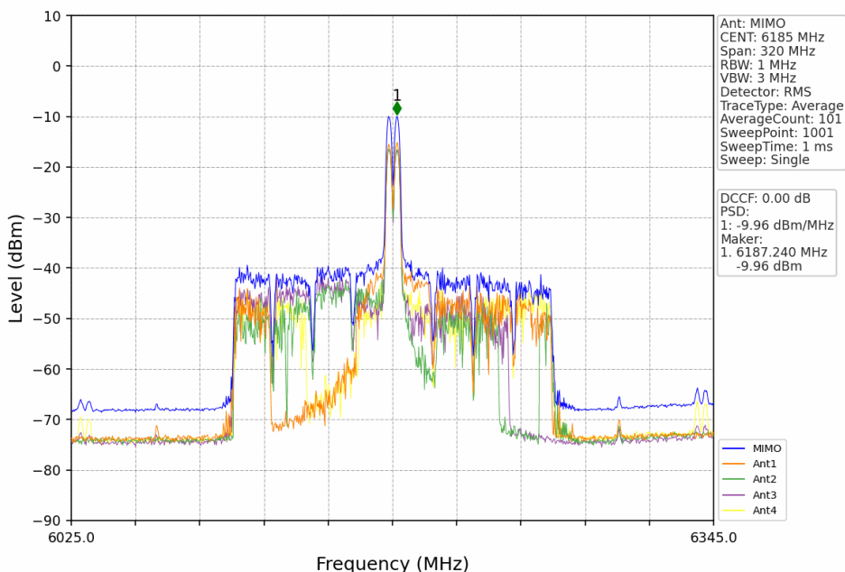
802.11ax(HEW160) MCH 6185MHz RU52+26 Mid MIMO NTN
