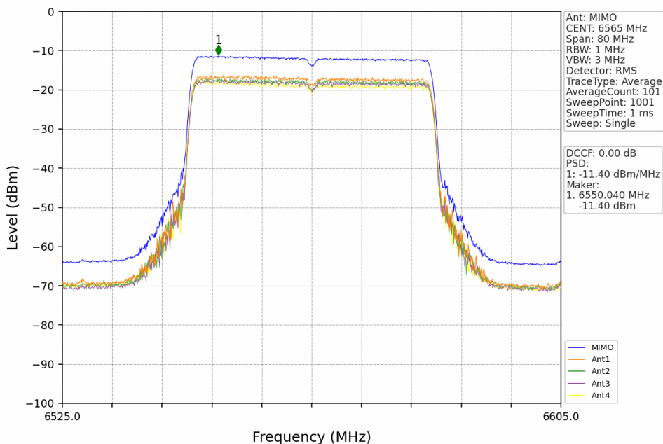
802.11ax(HEW40) LCH 6565MHz RU484 Left MIMO NTN
