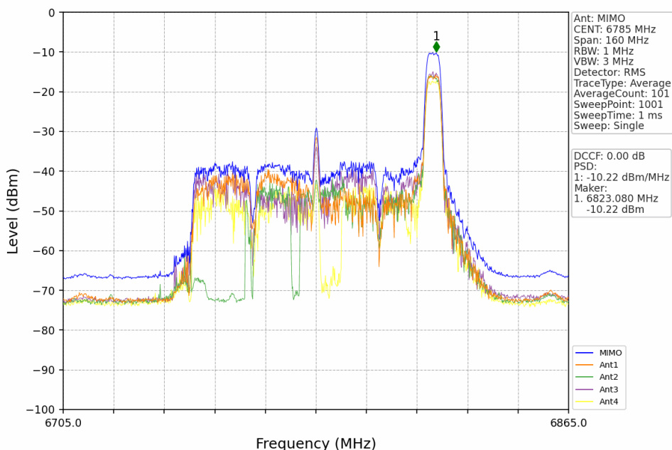
802.11ax(HEW80) HCH 6785MHz RU52+26 Right MIMO NTN
