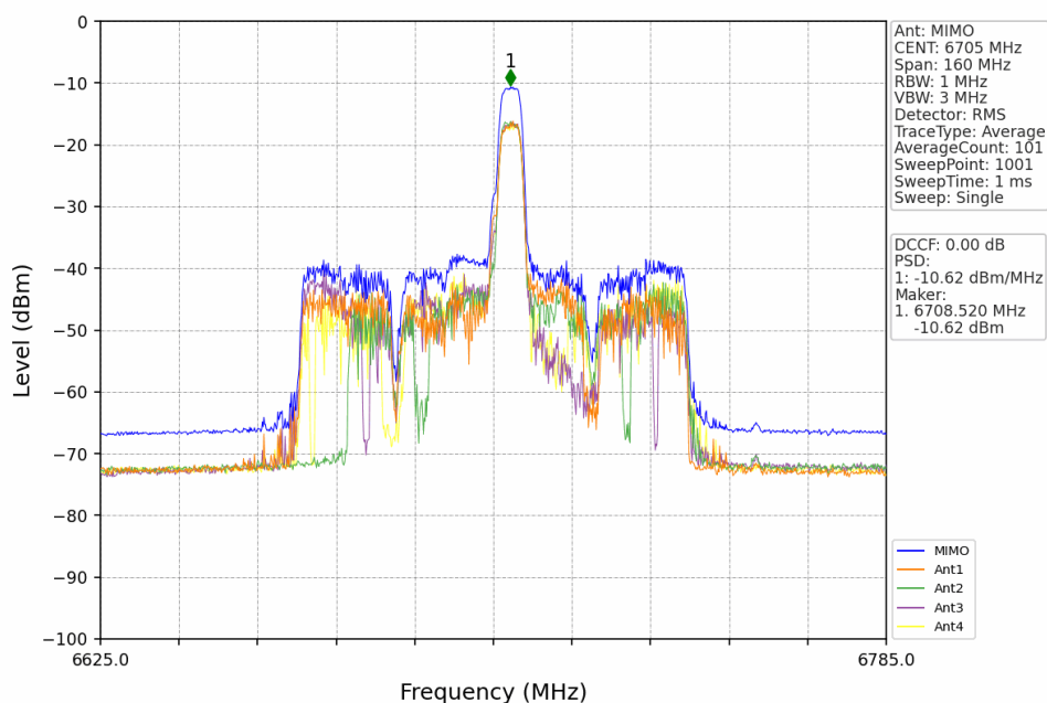
802.11ax(HEW80) MCH 6705MHz RU52 Mid MIMO NTN
