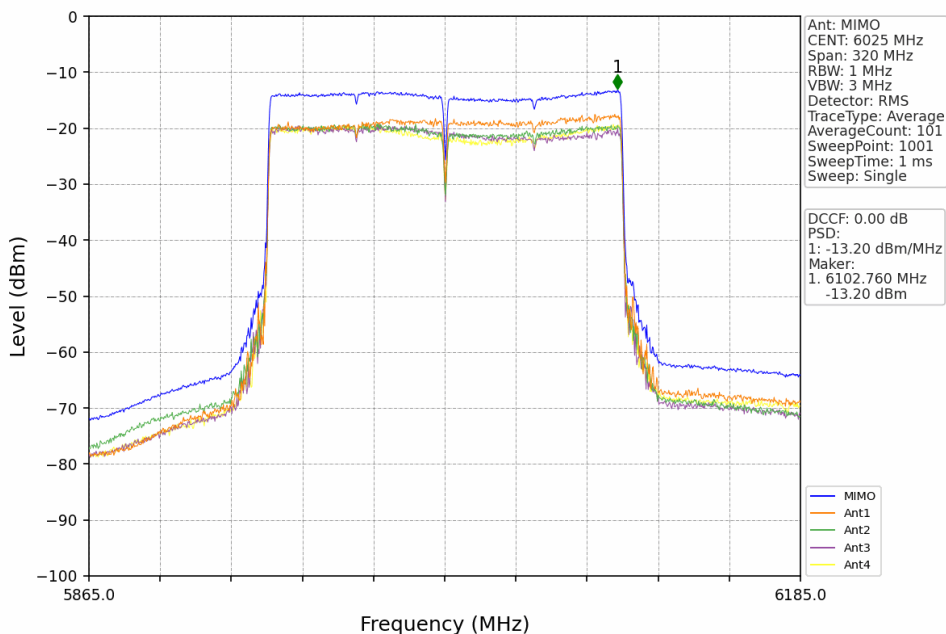
802.11ax(HEW160) LCH 6025MHz 2xRU996 Left MIMO NTNV
