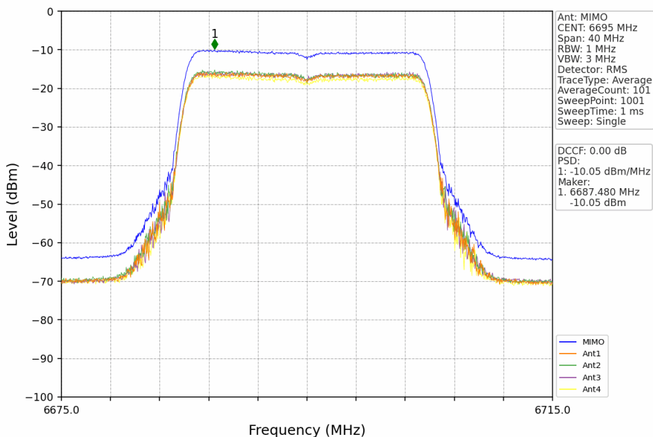
802.11ax(HEW20) MCH 6695MHz RU242 Left MIMO NTN
