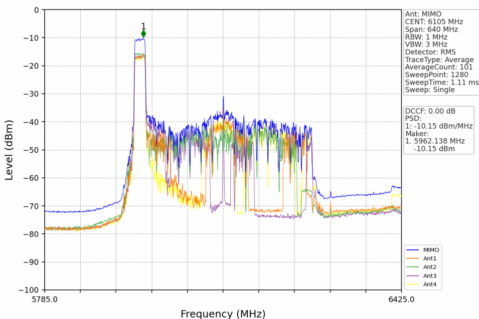
802.11be(EHT320)_LCH_6105MHz_RU52+26_Left_MIMO_NTNV
