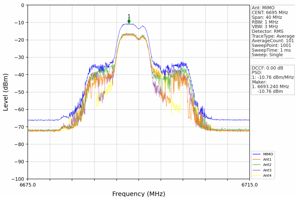
802.11be(EHT20)_MCH_6695MHz_RU52_Mid_MIMO_NTNV
