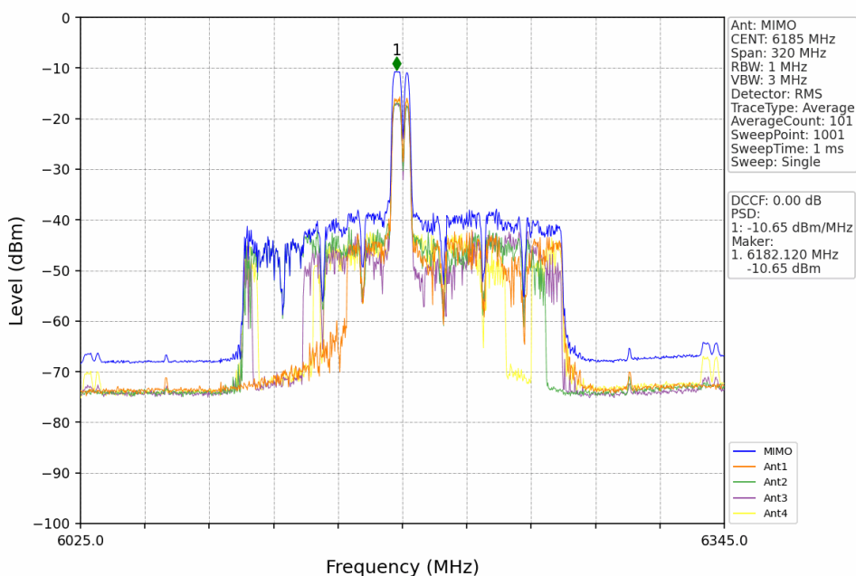
802.11be(EHT160)_MCH_6185MHz_RU52+26_Mid_MIMO_NTNV
