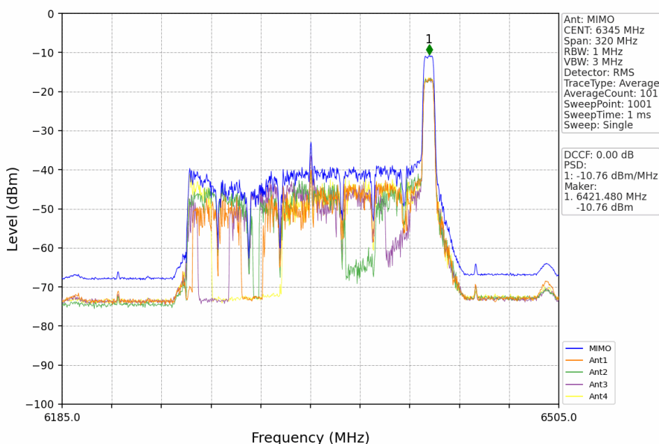
802.11be(EHT160)_HCH_6345MHz_2xRU996_Left_MIMO_NTNV
