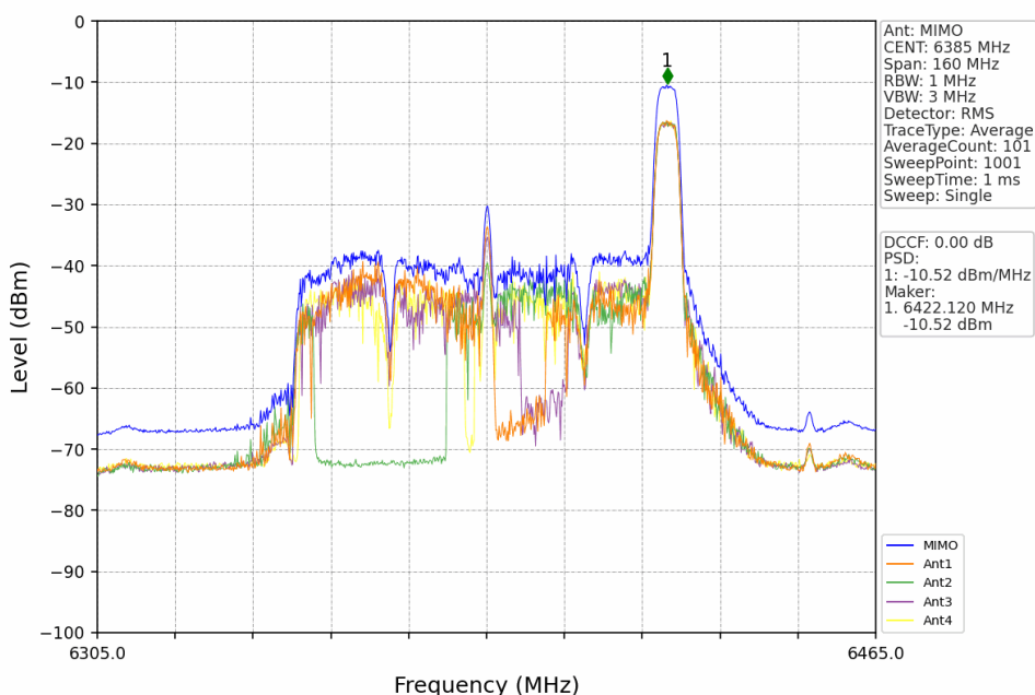
802.11be(EHT80)_HCH_6385MHz_RU52+26_Right_MIMO_NTNV
