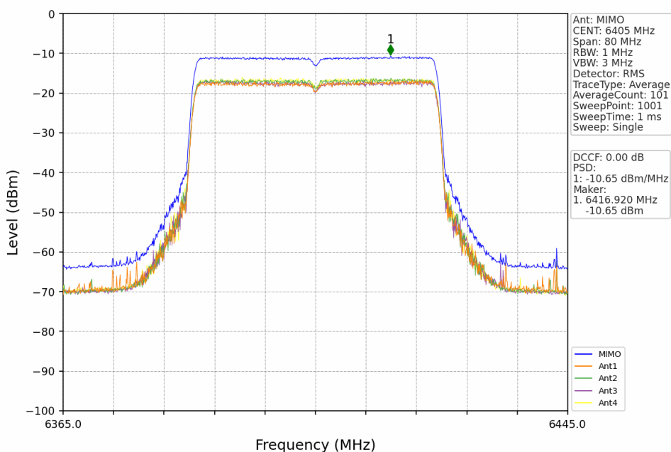
802.11be(EHT40)_HCH_6405MHz_RU484_Left_MIMO_NTNV
