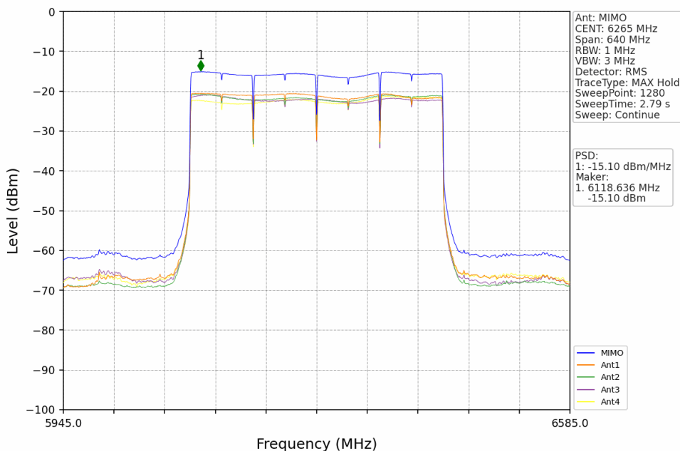
802.11be(EHT320)_HCH_6265MHz_4xRU996_Left_MIMO_NTNV
