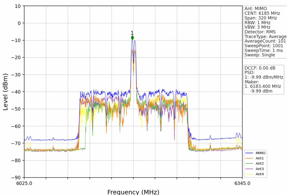
802.11be(EHT160)_MCH_6185MHz_RU52+26_Mid_MIMO_NTNV
