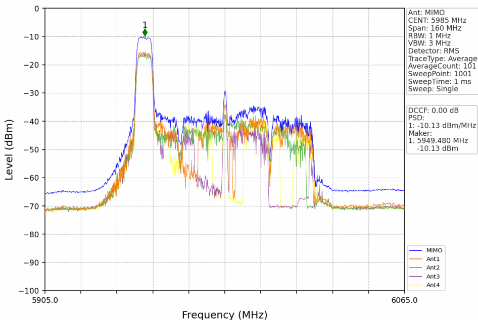
802.11be(EHT80)_LCH_5985MHz_RU52+26_Left_MIMO_NTNV
