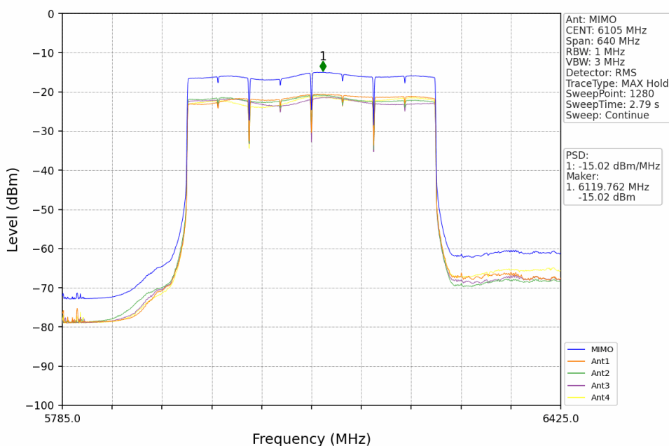
802.11be(EHT320)_LCH_6105MHz_4xRU996_Left_MIMO_NTNV
