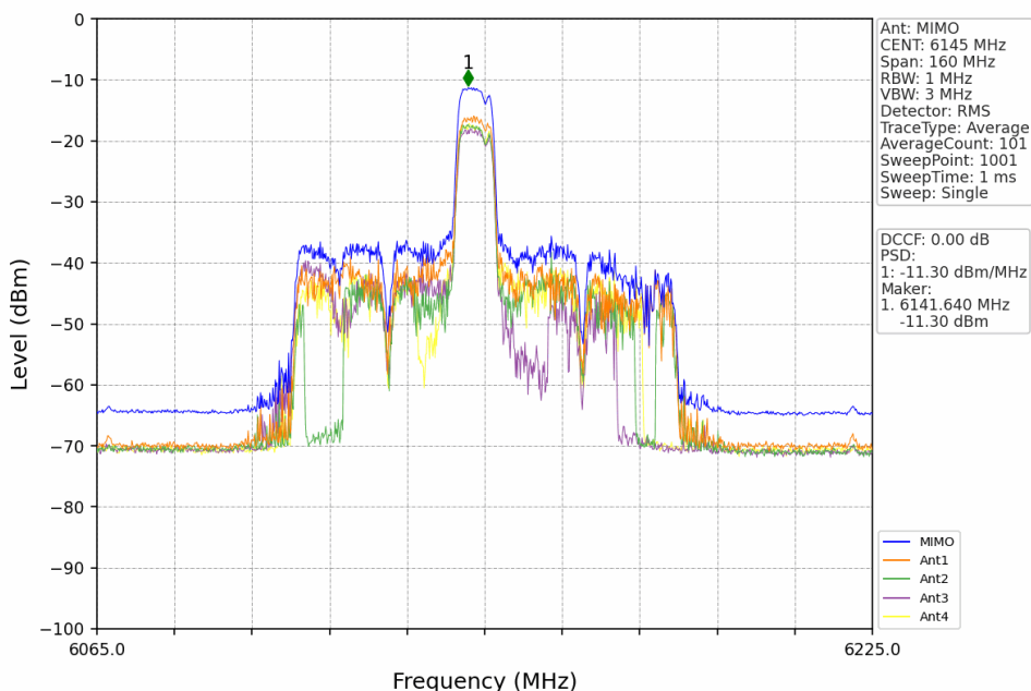
802.11be(EHT80)_MCH_6145MHz_RU996_Left_MIMO_NTNV
