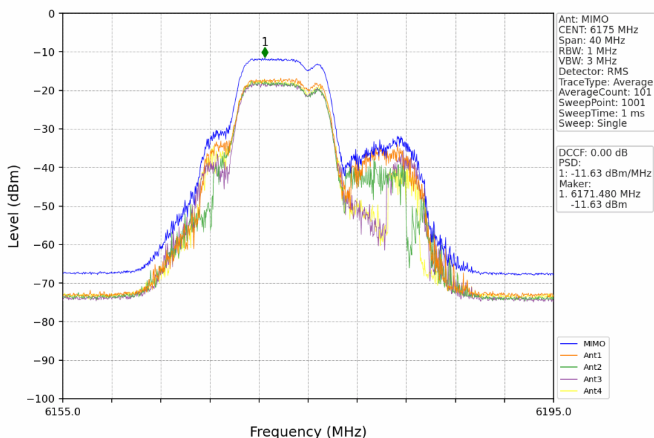
802.11be(EHT20)_MCH_6175MHz_RU242_Left_MIMO_NTNV
