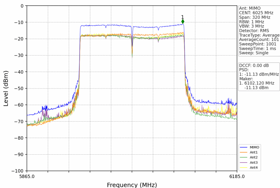
802.11be(EHT160)_LCH_6025MHz_2xRU996_Left_MIMO_NTNV
