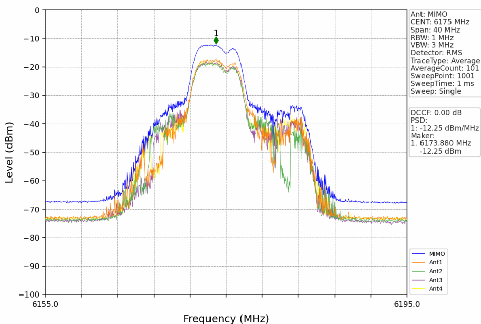
802.11be(EHT20)_MCH_6175MHz_RU52_Mid_MIMO_NTNV
