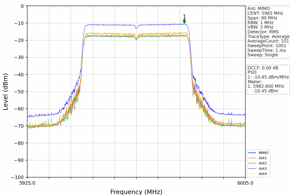
802.11be(EHT40)_LCH_5965MHz_RU484_Left_MIMO_NTNV
