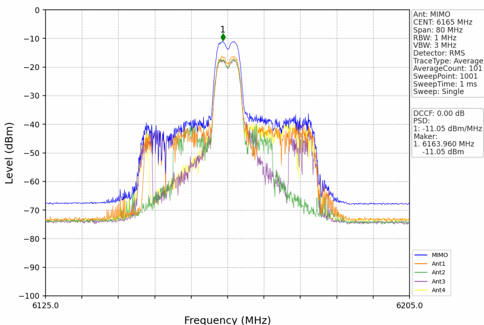
802.11be(EHT40)_MCH_6165MHz_RU52+26_Mid_MIMO_NTNV
