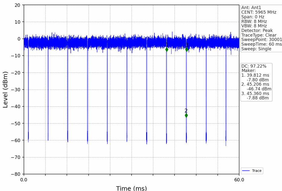
802.11be(EHT40)_LCH_5965MHz_RU484_Left_Ant1_NTNV
