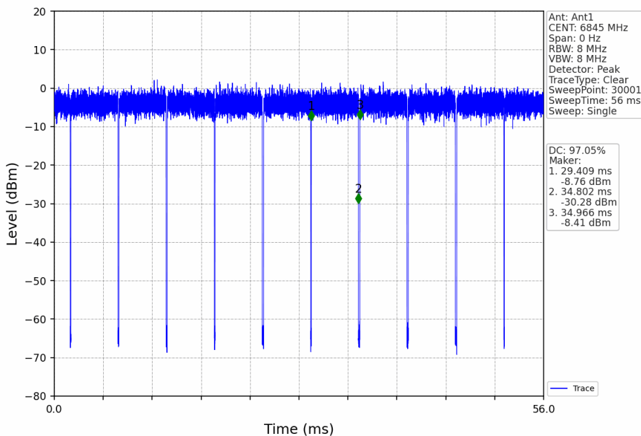
802.11be(EHT40)_HCH_6845MHz_RU484_Left_Ant1_NTNV
