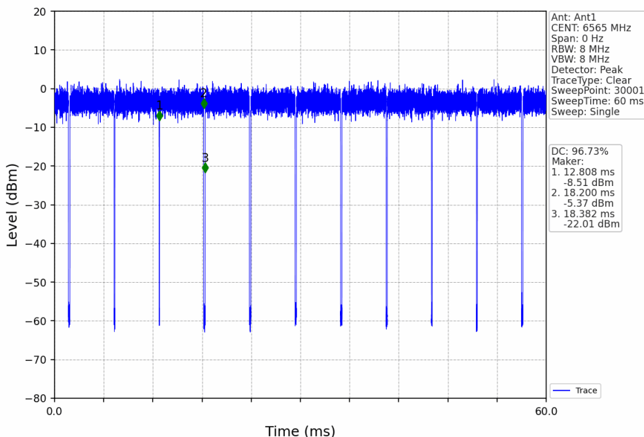
802.11be(EHT40)_LCH_6565MHz_RU484_Left_Ant1_NTNV
