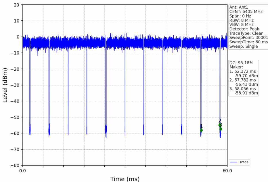
802.11be(EHT40)_HCH_6405MHz_RU484_Left_Ant1_NTNV
