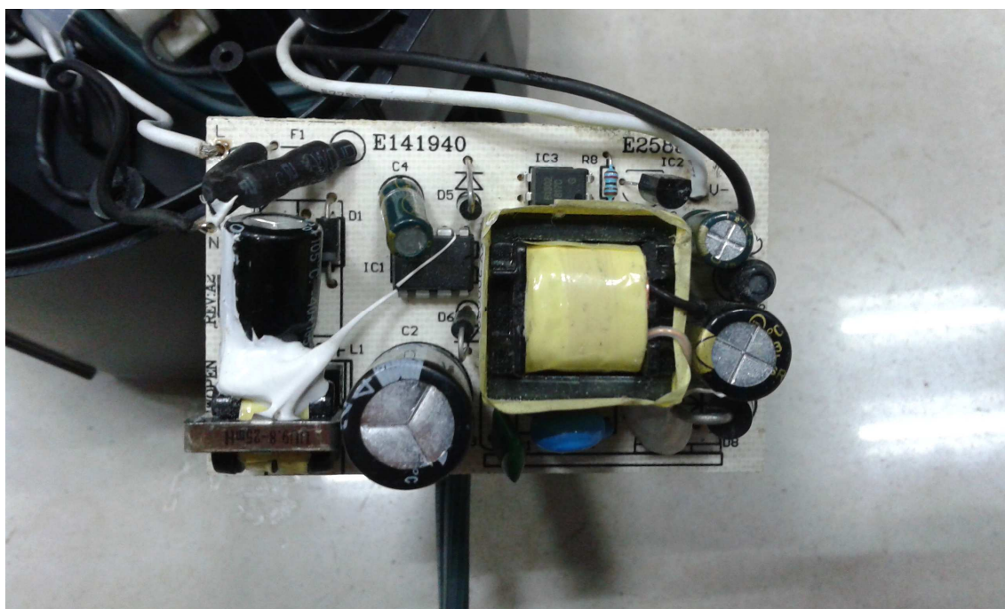
Adapter for MTS810-29V
