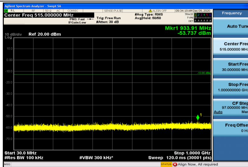
Band66-20MHz-QPSK-132572-1RB#0-30~1000MHz
