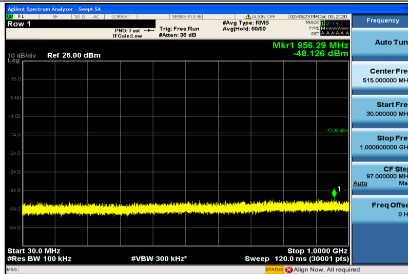
Band2-20MHz-16QAM-18700-1RB#0-30~1000MHz
