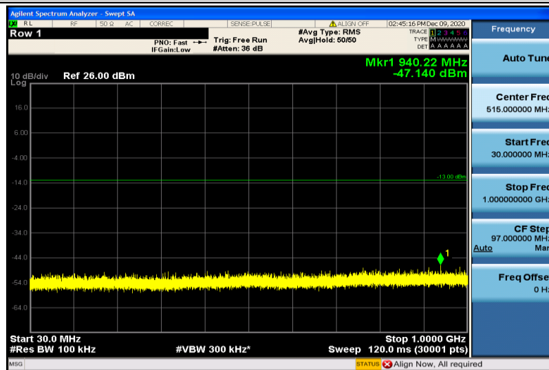
Band2-20MHz-QPSK-19100-1RB#0-30~1000MHz
