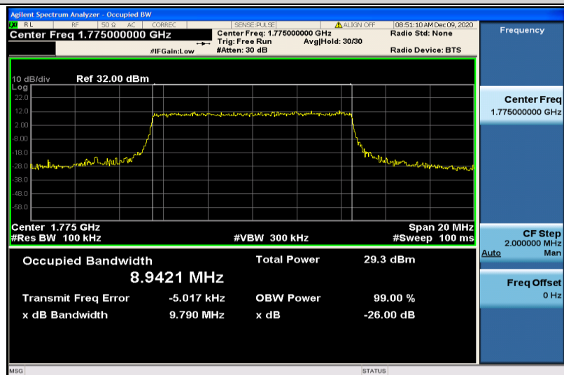
Band66-10MHz-QPSK-132622-50RB#0-8.9421
