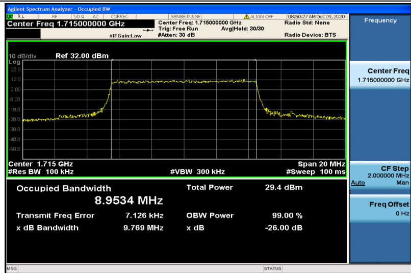
Band66-10MHz-QPSK-132022-50RB#0-8.9534
