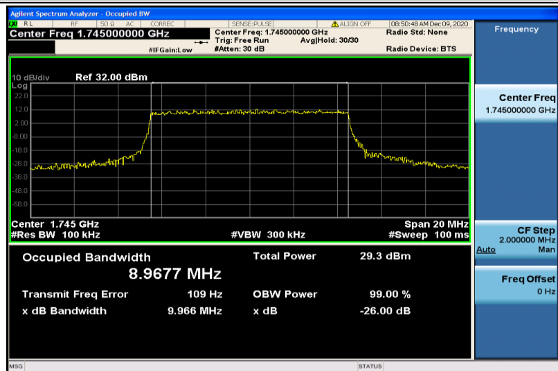
Band66-10MHz-QPSK-132322-50RB#0-8.9677
