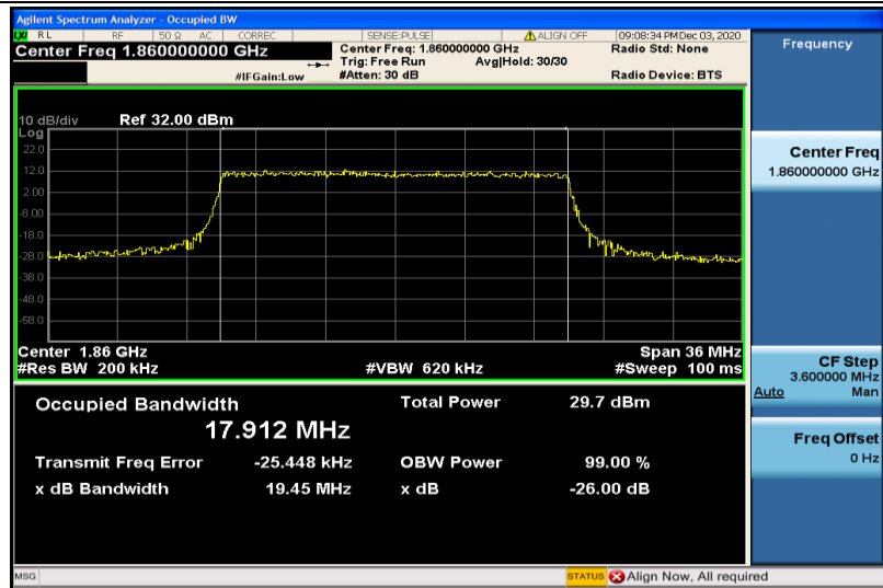
Band2-20MHz-QPSK-18700-100RB#0-17.912
