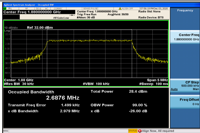
Band2-3MHz-QPSK-18900-15RB#0-2.6876
