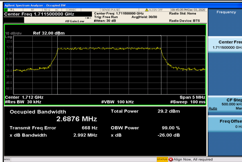
Band4-3MHz-QPSK-19965-15RB#0-2.6876
