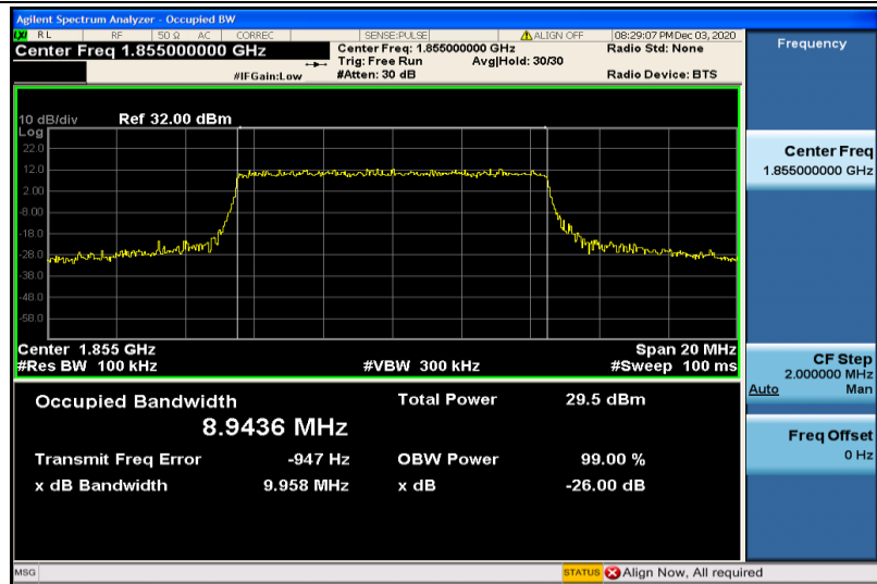
Band2-10MHz-QPSK-18650-50RB#0-8.9436
