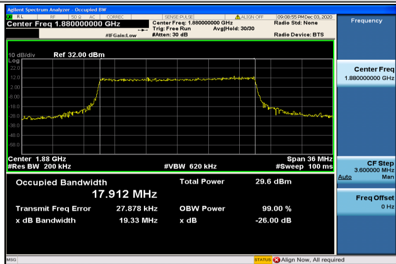
Band2-20MHz-QPSK-18900-100RB#0-17.912
