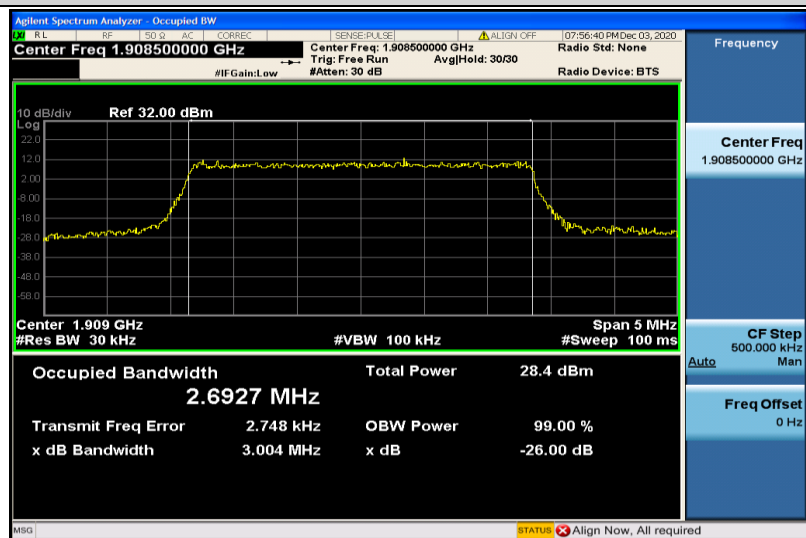
Band2-3MHz-QPSK-19185-15RB#0-2.6927
