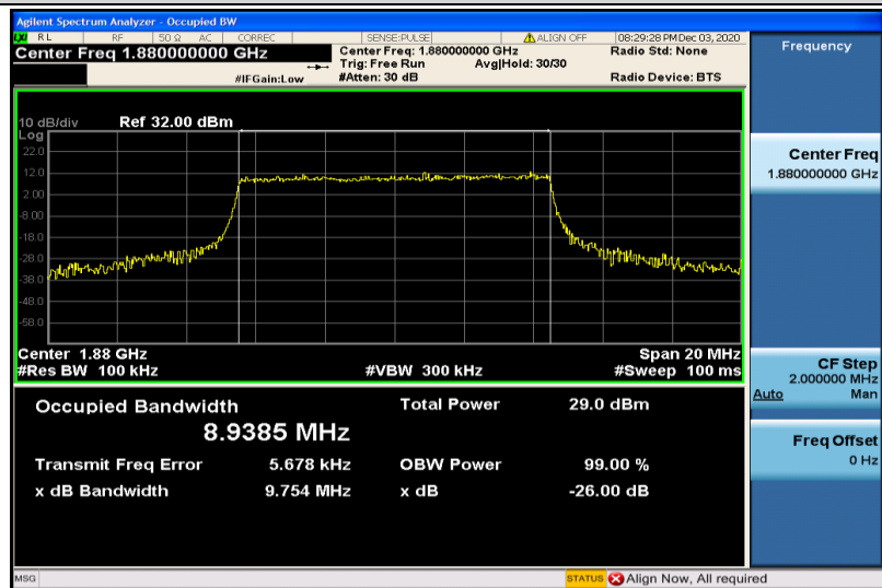
Band2-10MHz-QPSK-18900-50RB#0-8.9385
