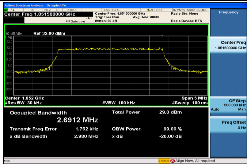
Band2-3MHz-QPSK-18615-15RB#0-2.6912
