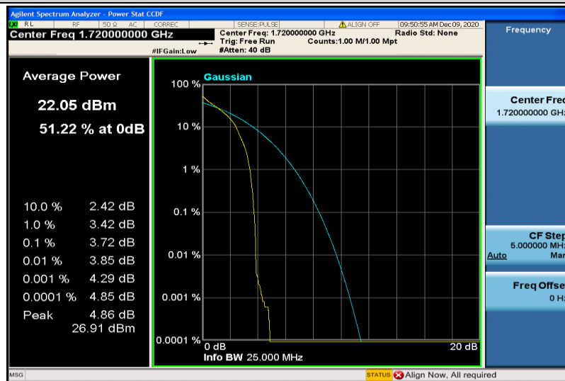
Band66-20MHz-QPSK-132072-1RB#0
