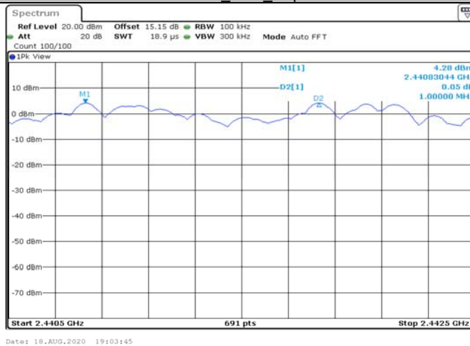
3DH1_Ant1_Hop
