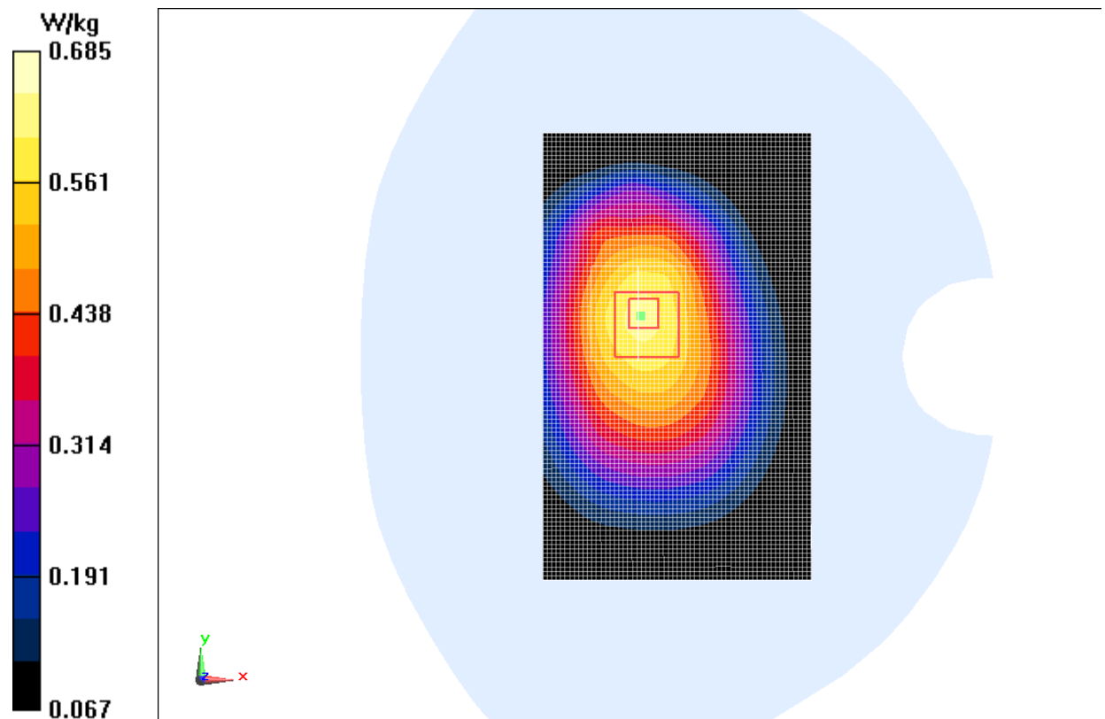
Fig.6 WCDMA 850 CH4182
