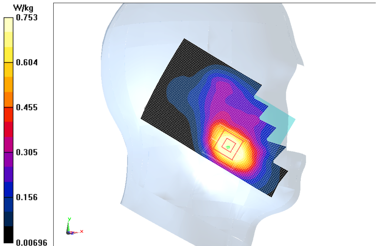
Fig.7 WCDMA1900 CH9538
