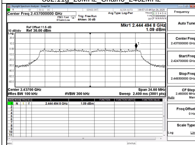
802.11g 20MHz Chain1 2437MHz
