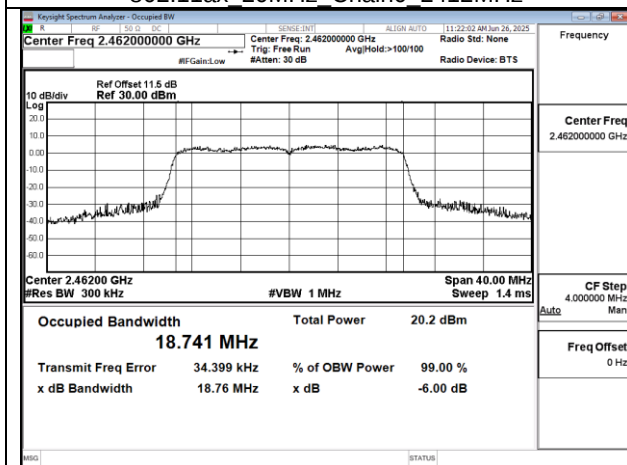
802.11ax 20MHz Chain0 2462MHz
