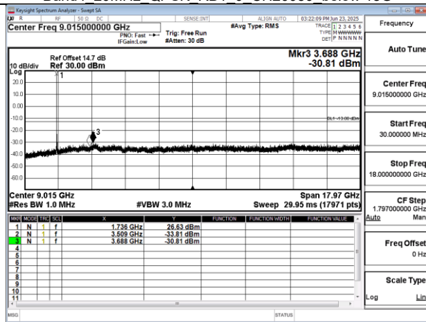
Band4 20MHz QPSK RB1 0 CH20300 below 18G
