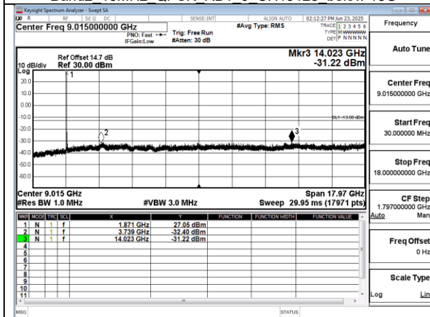
Band2 20MHz QPSK RB1 0 CH18900 below 18G
