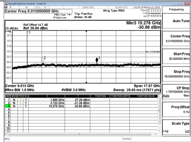
Band2 1.4MHz QPSK RB1 0 CH18900 below 18G
