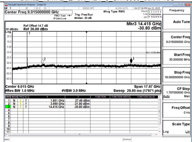
Band2 20MHz QPSK RB1 0 CH18700 below 18G
