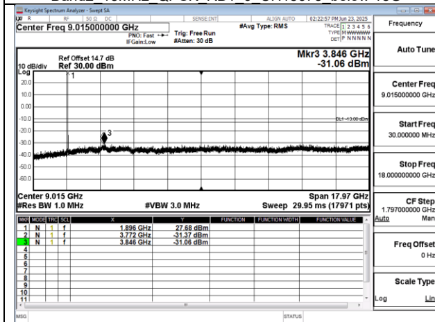
Band2 15MHz QPSK RB1 0 CH19125 below 18G
