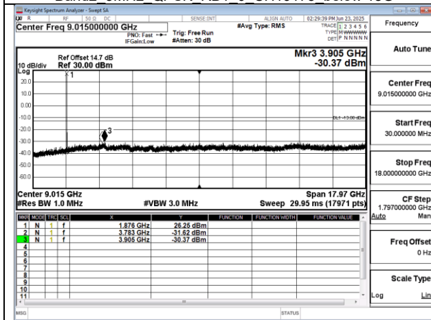
Band2 10MHz QPSK RB1 0 CH18900 below 18G
