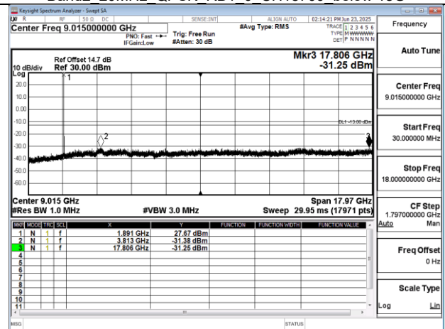
Band2 20MHz QPSK RB1 0 CH19100 below 18G
