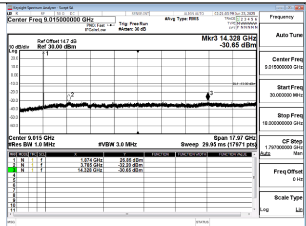
Band2 15MHz QPSK RB1 0 CH18900 below 18G
