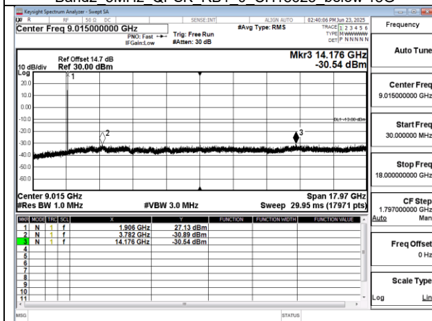
Band2 5MHz QPSK RB1 0 CH19175 below 18G
