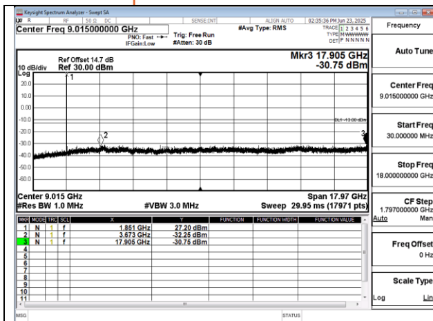
Band2 5MHz QPSK RB1 0 CH18625 below 18G
