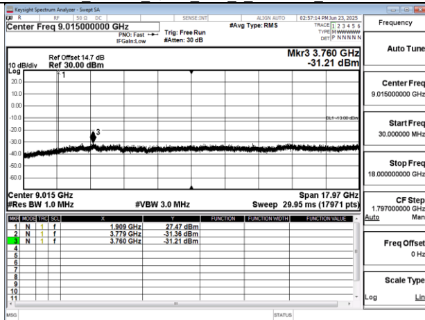
Band2 1.4MHz QPSK RB1 0 CH19193 below 18G
