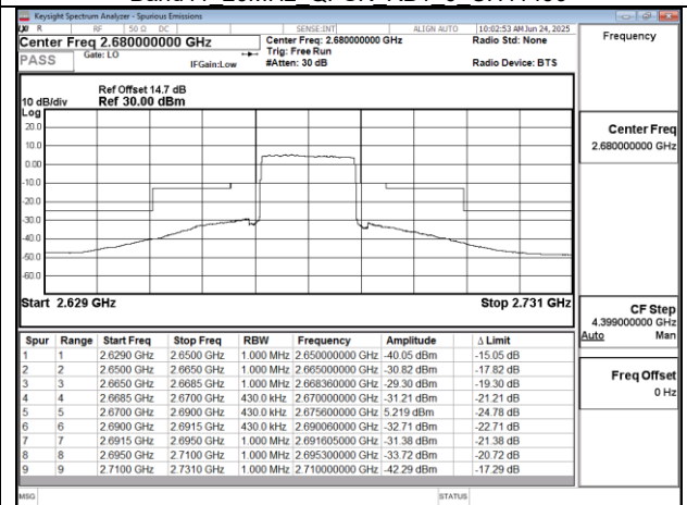
Band41 20MHz QPSK RB100 0 CH41490
