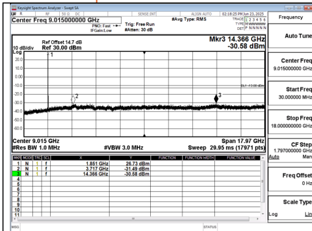
Band2 15MHz QPSK RB1 0 CH18675 below 18G
