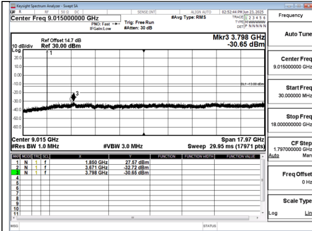
Band2 1.4MHz QPSK RB1 0 CH18607 below 18G
