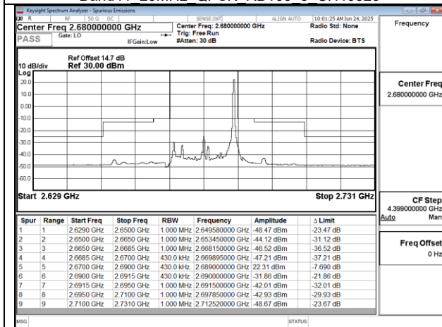
Band41 20MHz QPSK RB1 99 CH41490
