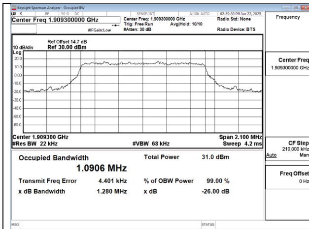
Band2 1.4MHz 16QAM RB6 0 CH19193
