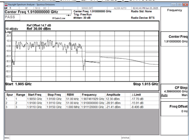
Band2 5MHz QPSK RB25 0 CH19175
