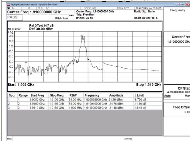
Band2 5MHz QPSK RB1 24 CH19175
