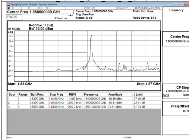
Band2 20MHz QPSK RB1 0 CH18700
