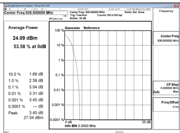
WCDMA B5 Mid CH4183-836.6
