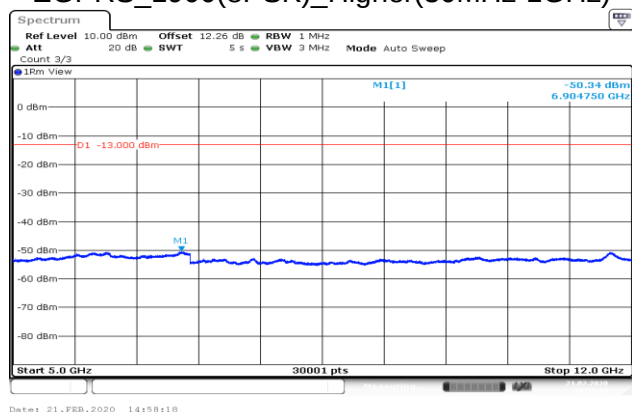
EGPRS_1900(8PSK)_Higher(5GHz-12GHz)
