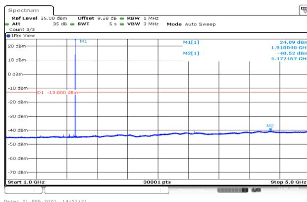
EGPRS_1900(8PSK)_Higher(1GHz-5GHz)
