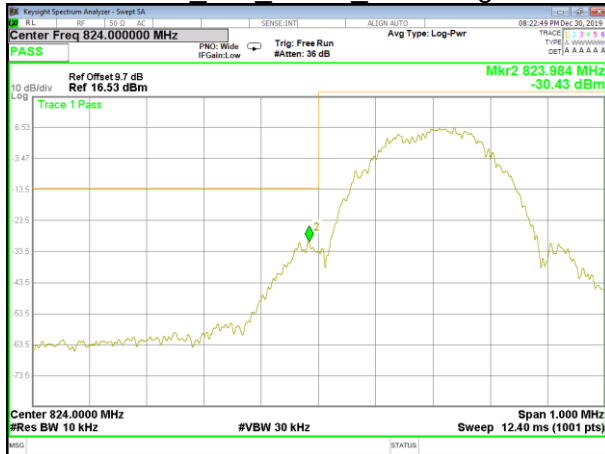
EGPRS_850(8PSK)_Lower_Band edge
