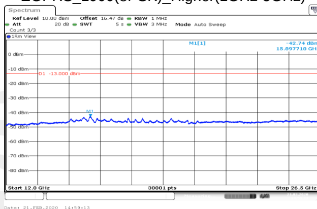
EGPRS_1900(8PSK)_Higher(12GHz-26.5GHz)
