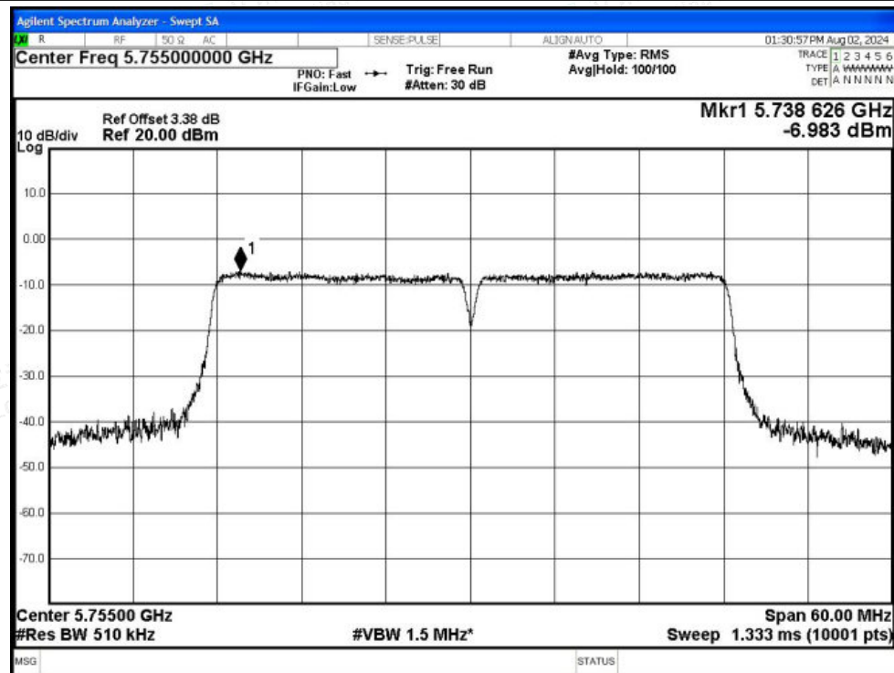
PSD NVNT n40 5755MHz Ant0
