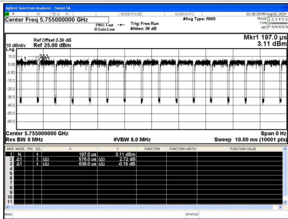
Duty Cycle NVNT n40 5755MHz Ant0
