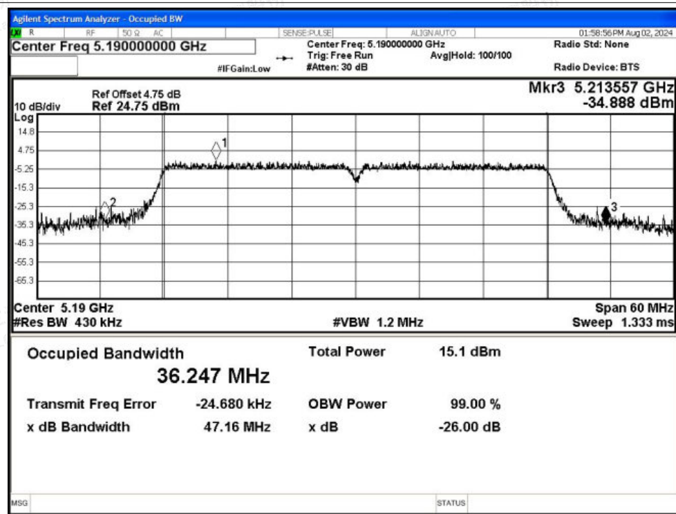
-26dB Bandwidth NVNT n40 5190MHz Ant0
